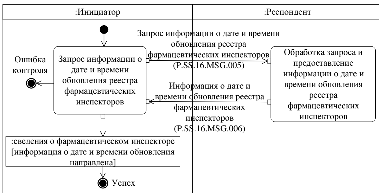
Рис. 7. Схема выполнения транзакции общего процесса «Получение информации о дате и времени обновления реестра фармацевтических инспекторов» (P.SS.16.TRN.004)
