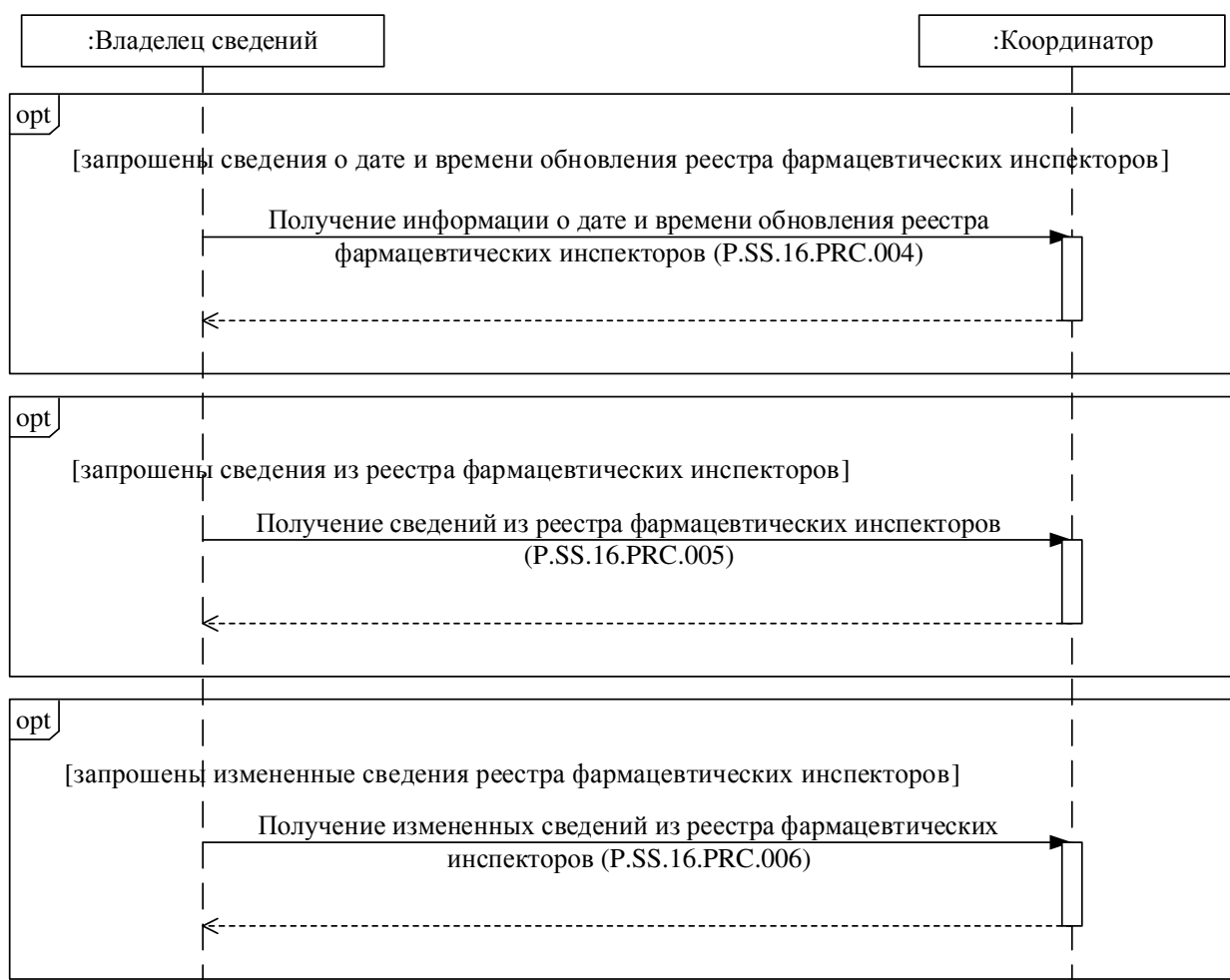
Рис. 3. Схема выполнения транзакций общего процесса при получении сведений из реестра фармацевтических инспекторов по запросу уполномоченных органов
