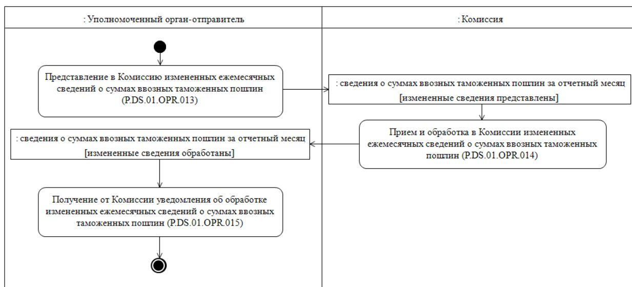
Рис. 5. Схема выполнения процедуры «Представление в Комиссию измененных ежемесячных сведений о суммах ввозных таможенных пошлин» (P.DS.01.PRC.005)
