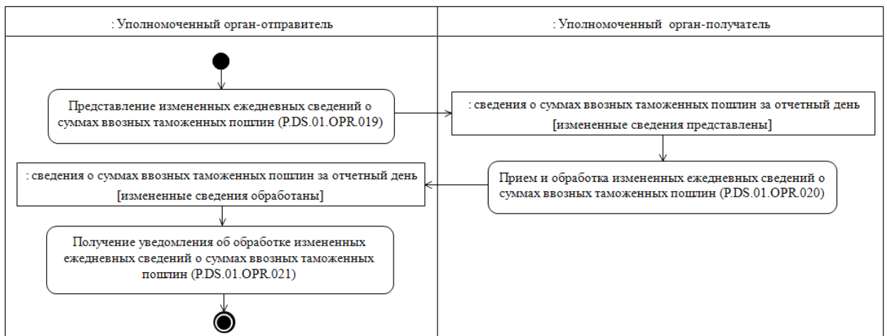
Рис. 6. Схема выполнения процедуры «Представление в уполномоченные органы измененных ежедневных сведений о суммах ввозных таможенных пошлин» (P.DS.01.PRC.007)
