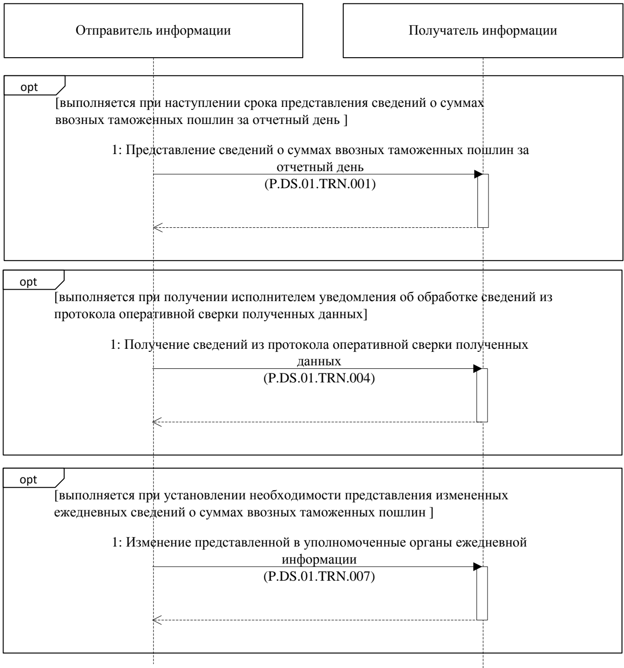
Рис. 2. Схема выполнения транзакций общего процесса при представлении сведений уполномоченными органами друг другу
