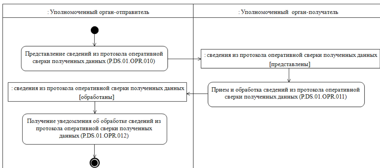
Рис. 4. Схема выполнения процедуры «Представление уполномоченными органами друг другу сведений из протокола оперативной сверки полученных данных» (P.DS.01.PRC.004)
