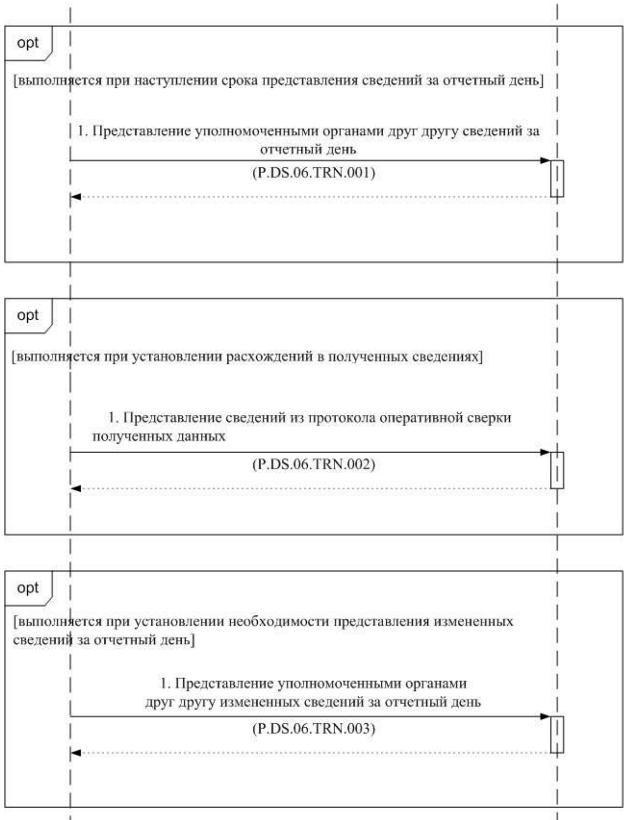
Рис. 2. Схема выполнения транзакций общего процесса при представлении сведений уполномоченными органами друг другу
