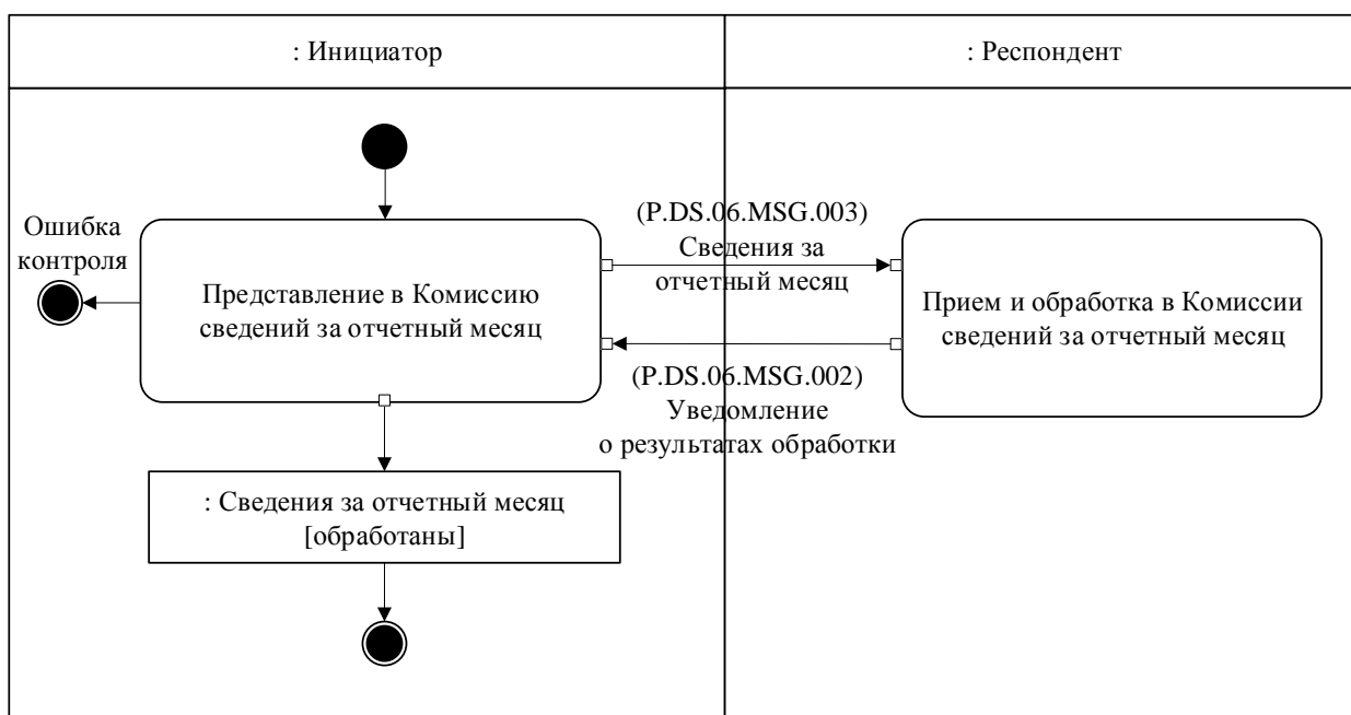
Рис. 3. Схема выполнения транзакции общего процесса «Представление уполномоченными органами в Комиссию сведений за отчетный месяц» (P.DS.06.TRN.004)
