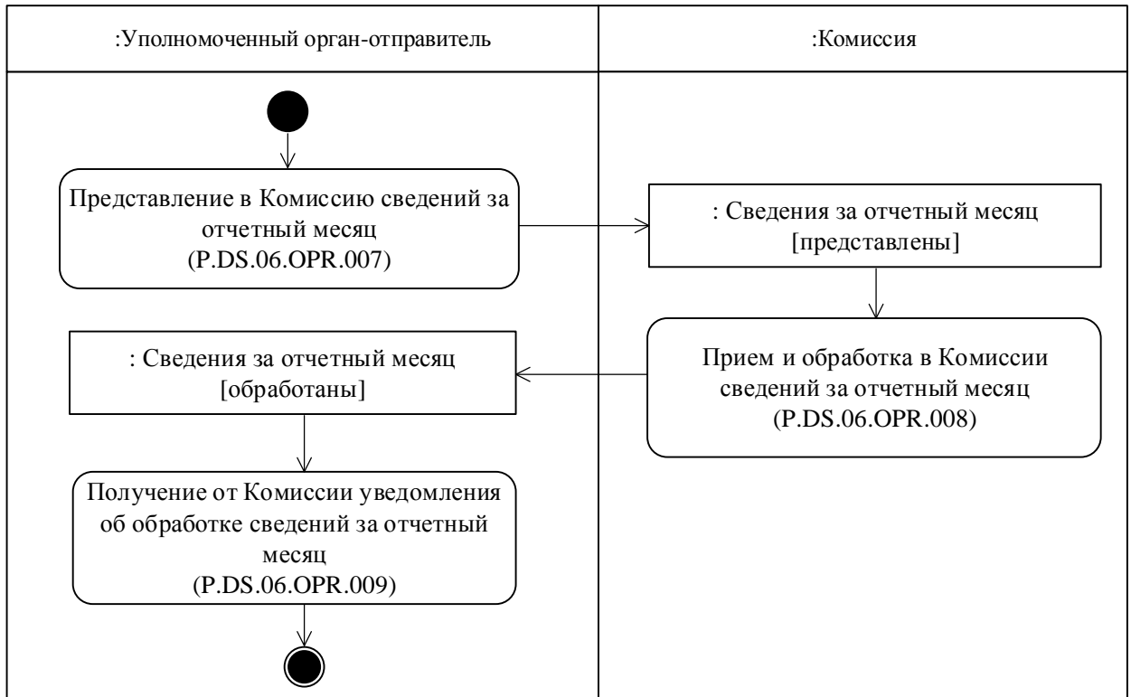
Рис. 3. Схема выполнения процедуры «Представление уполномоченными органами в Комиссию сведений за отчетный месяц» (P.DS.06.PRC.002)
