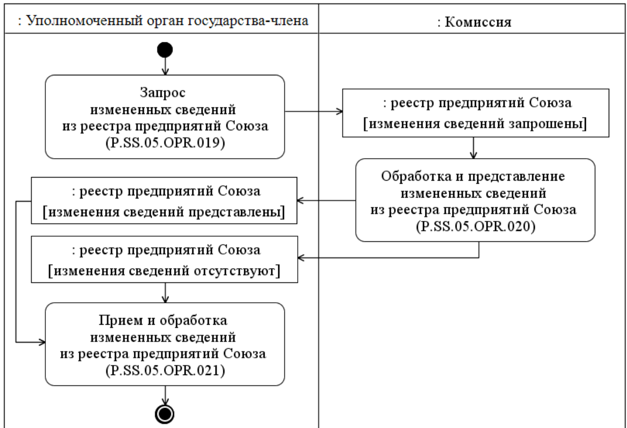
Рис. 9. Схема выполнения процедуры «Получение измененных сведений из реестра предприятий Союза» (P.SS.05.PRC.006)
