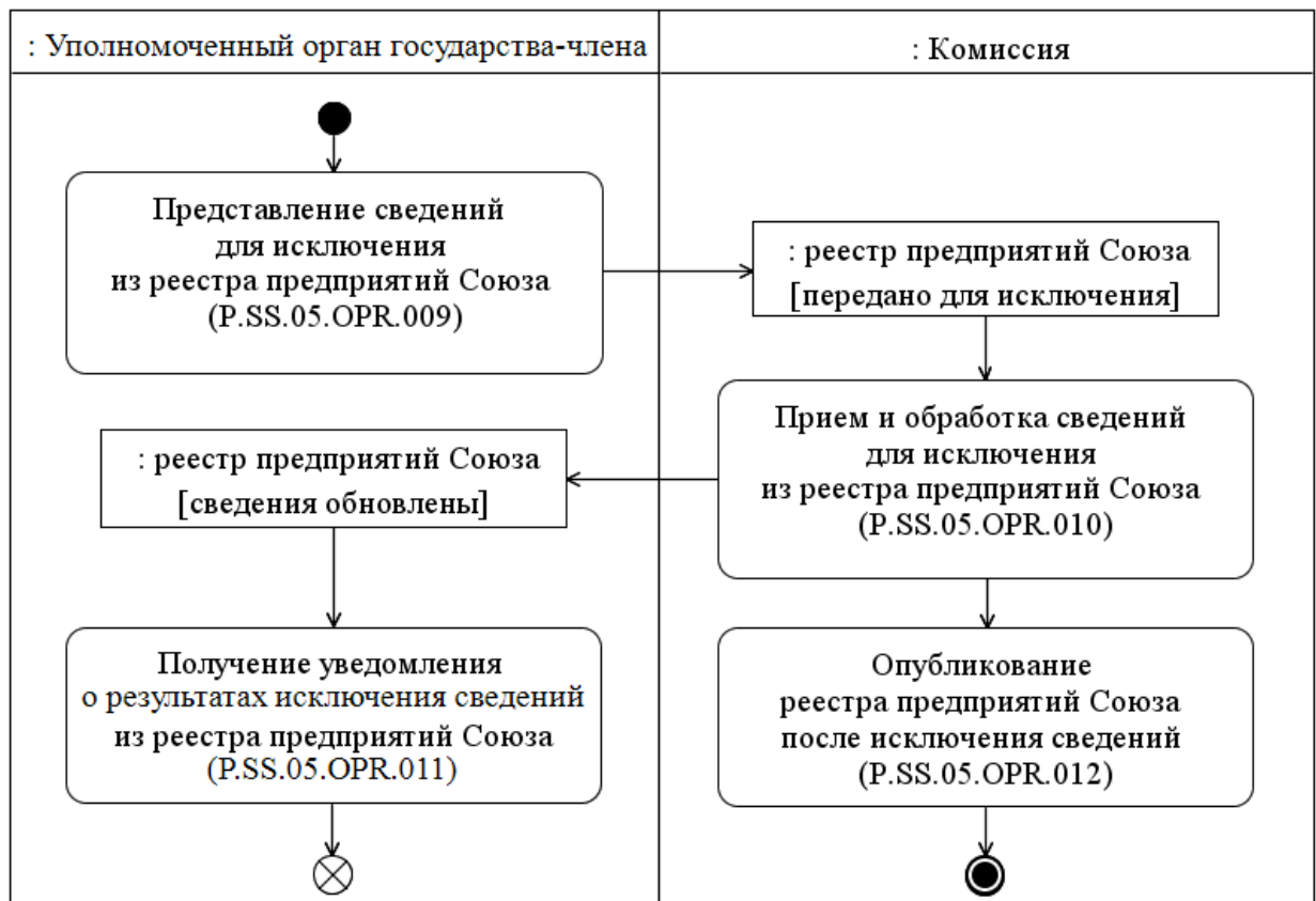
Рис. 6. Схема выполнения процедуры «Исключение сведений из реестра предприятий Союза» (P.SS.05.PRC.003)
