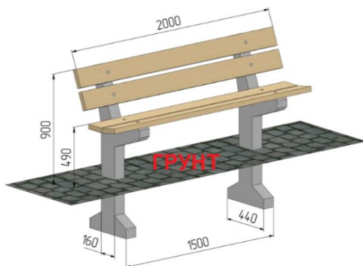
Рисунок 1 – Скамья уличная вкапываемая
