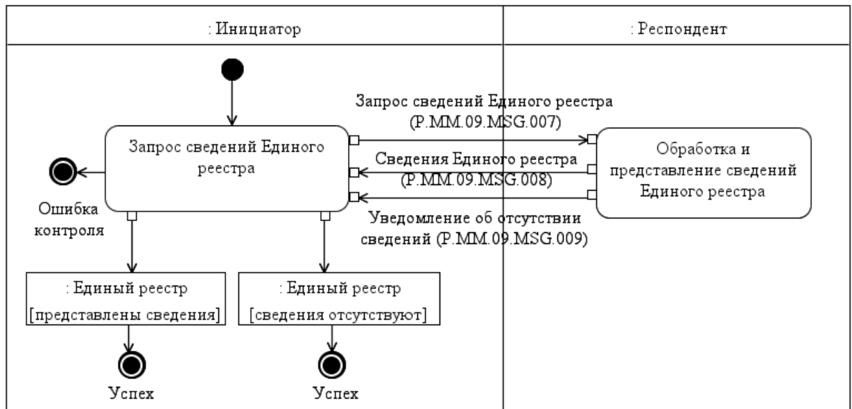
Рис. 8. Схема выполнения транзакции общего процесса «Получение сведений из Единого реестра» (P.MM.09.TRN.005)
