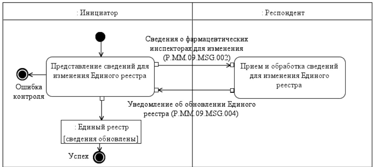
Рис. 5. Схема выполнения транзакции общего процесса «Передача сведений для изменения в Едином реестре» (P.MM.09.TRN.002)
