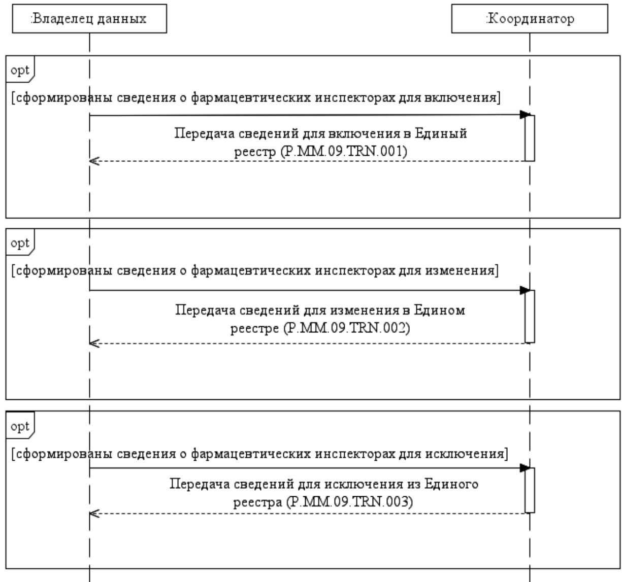
Рис. 2. Схема выполнения транзакций общего процесса при формировании Единого реестра
