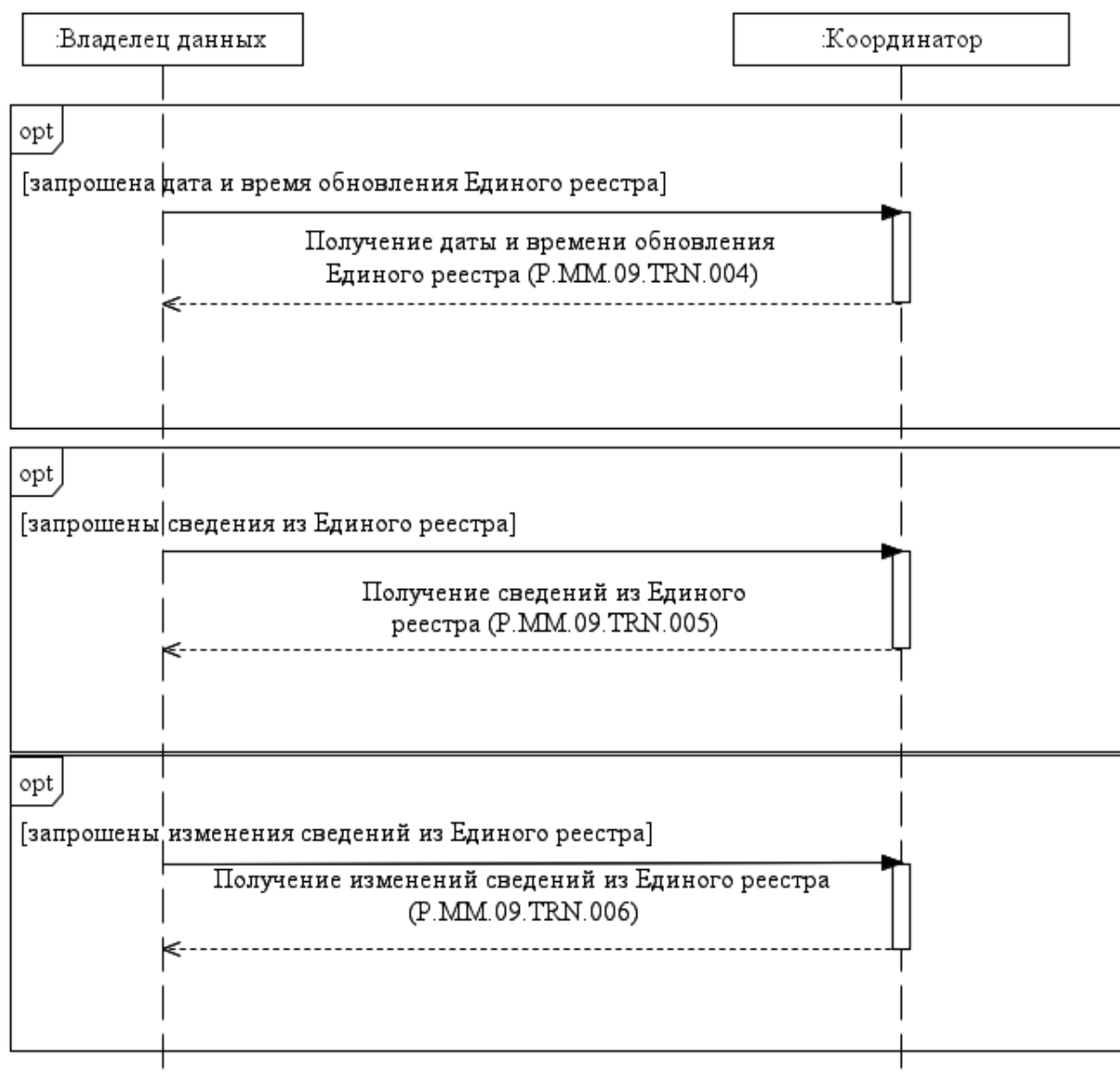
Рис. 3. Схема выполнения транзакций общего процесса при получении сведений из Единого реестра
