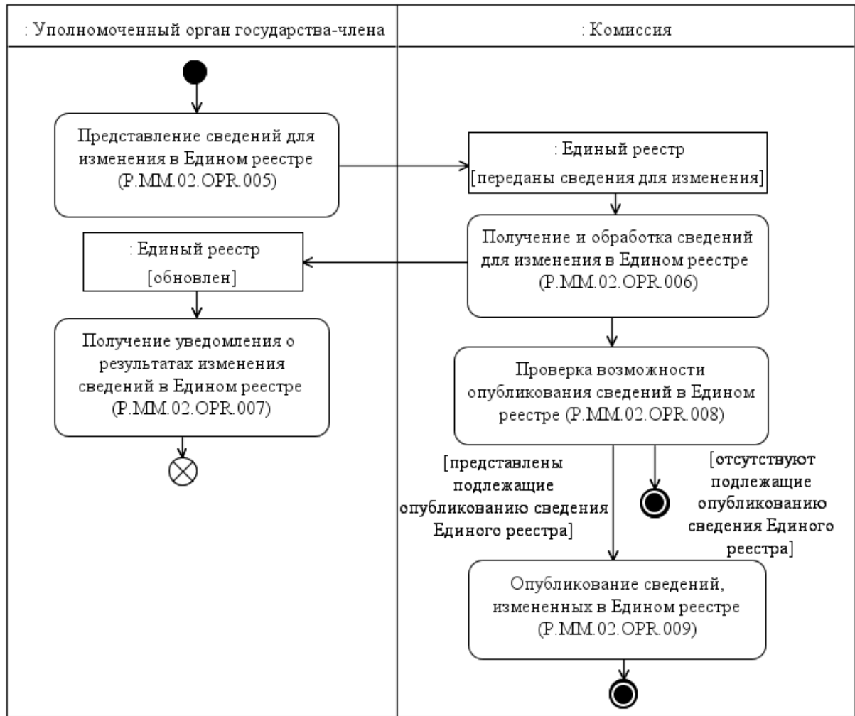
Рис. 5. Схема выполнения процедуры «Изменение сведений в Едином реестре» (P.MM.02.PRC.002)
