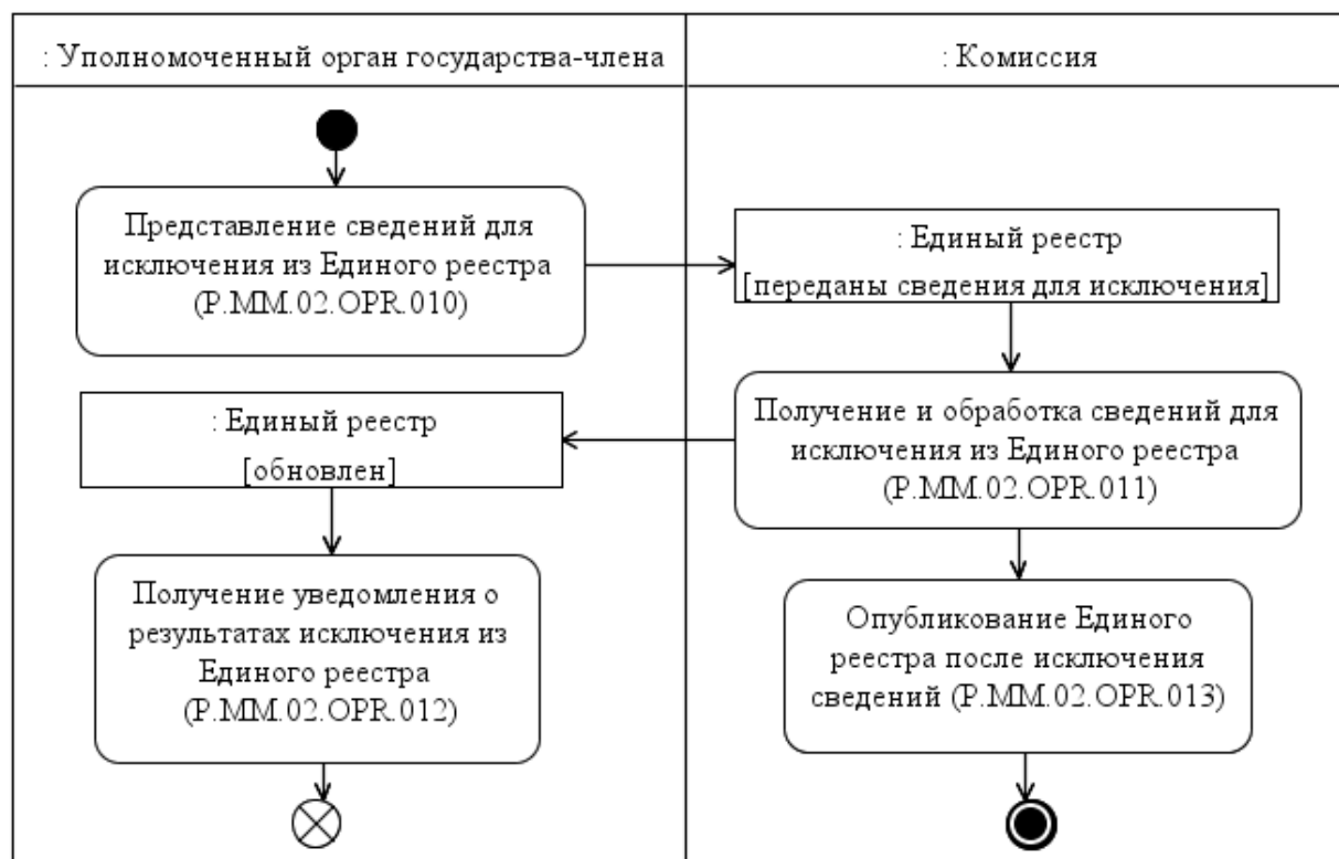
Рис. 6. Схема выполнения процедуры «Исключение сведений из Единого реестра» (P.MM.02.PRC.003)
