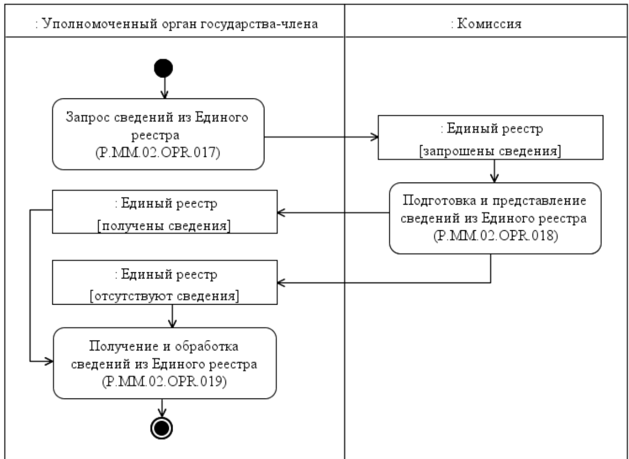
Рис. 8. Схема выполнения процедуры «Получение сведений из Единого реестра» (P.MM.02.PRC.005)
