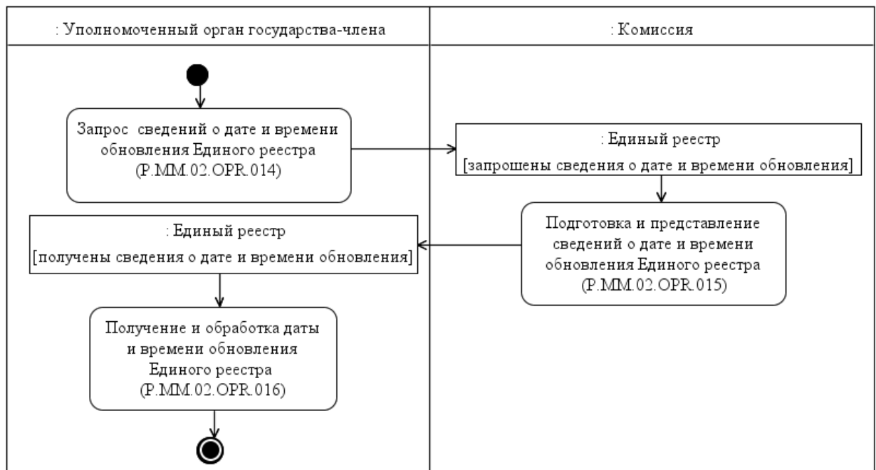
Рис. 7. Схема выполнения процедуры «Получение сведений о дате и времени обновления Единого реестра» (P.MM.02.PRC.004)
