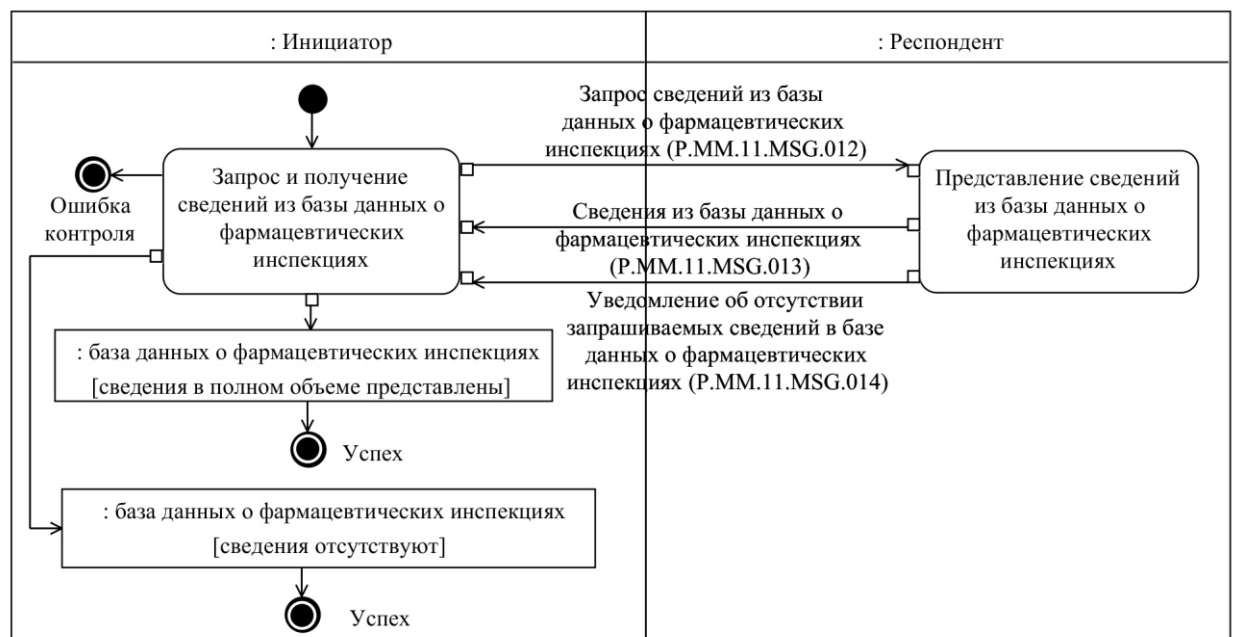
Рис. 11. Схема выполнения транзакции общего процесса «Получение сведений из базы данных о фармацевтических инспекциях» (P.MM.11.TRN.008)
