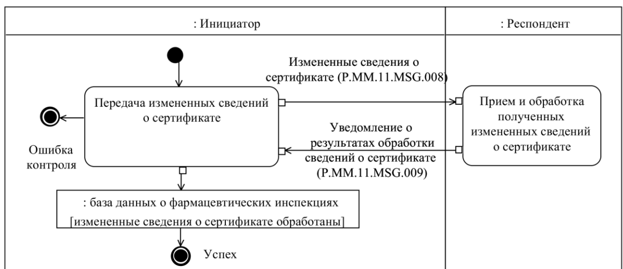
Рис. 9. Схема выполнения транзакции общего процесса «Представление измененных по результатам инспекции сведений о сертификате» (P.MM.11.TRN.006)
