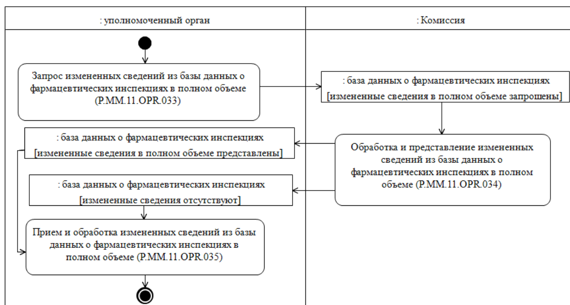
Рис. 15. Схема выполнения процедуры «Получение измененных сведений из базы данных о фармацевтических инспекциях в полном объеме» (P.MM.11.PRC.011)
