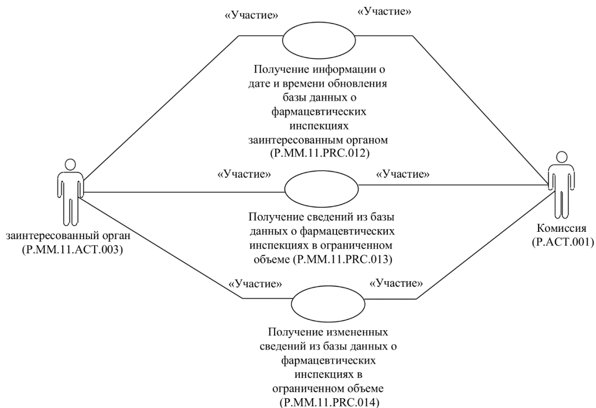
Рис. 4. Общая схема группы процедур представления сведений из базы данных о фармацевтических инспекциях в ограниченном объеме
