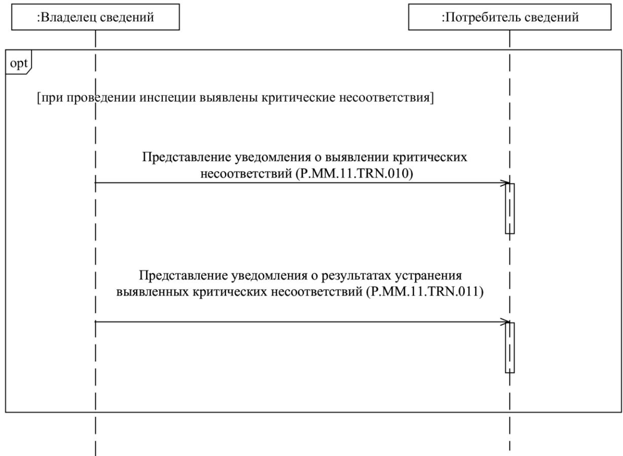
Рис. 2. Схема выполнения транзакций общего процесса при уведомлении о выявлении критических несоответствий и результатах их устранения
