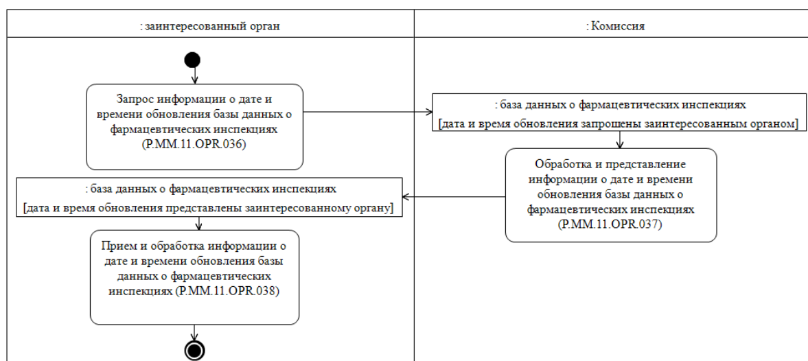
Рис. 17. Схема выполнения процедуры «Получение сведений из базы данных о фармацевтических инспекциях в ограниченном объеме» (P.MM.11.PRC.013)
