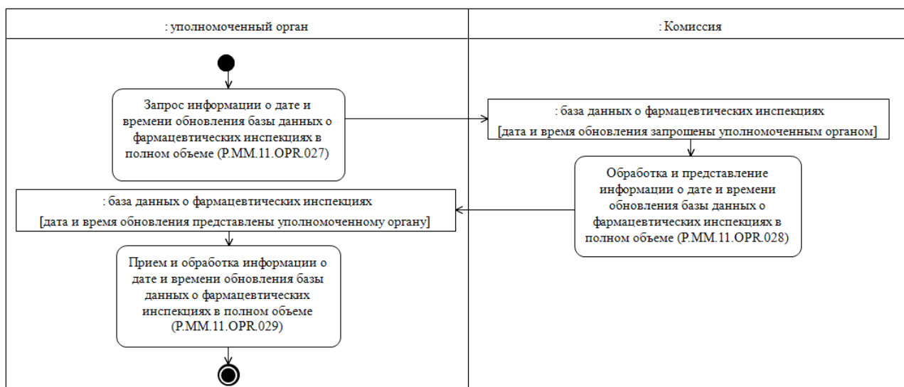
Рис. 13. Схема выполнения процедуры «Получение информации о дате и времени обновления базы данных о фармацевтических инспекциях уполномоченным органом» (P.MM.11.PRC.009)
