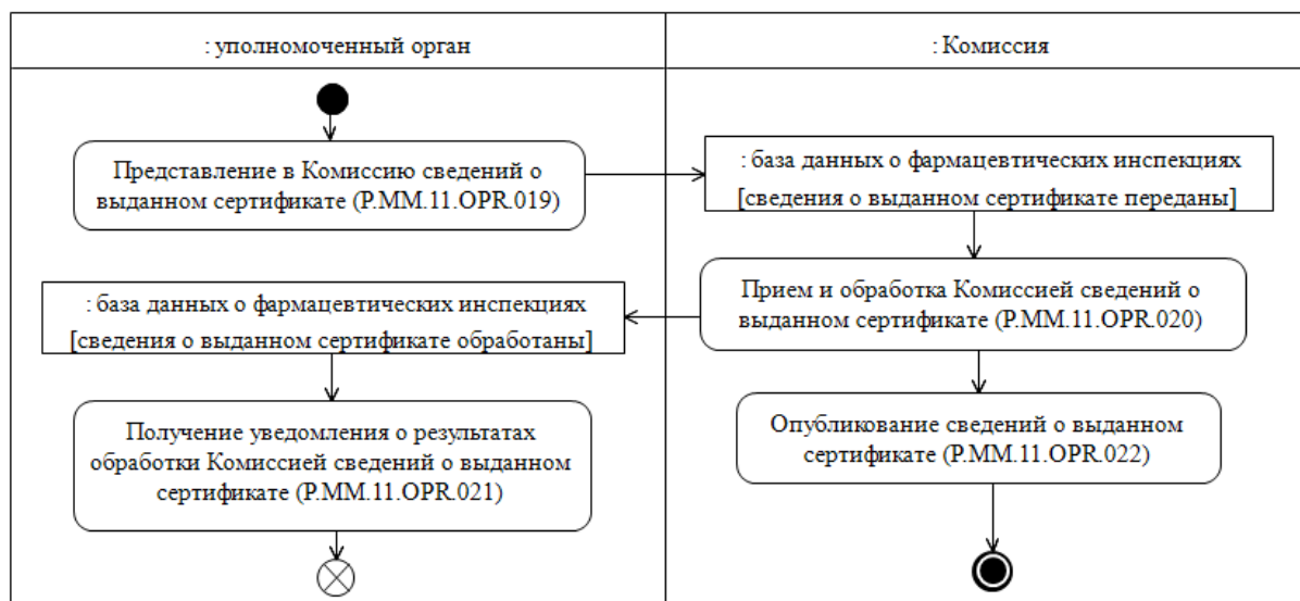
Рис. 11. Схема выполнения процедуры «Представление в Комиссию сведений о выданном по результатам фармацевтической инспекции сертификате» (P.MM.11.PRC.007)
