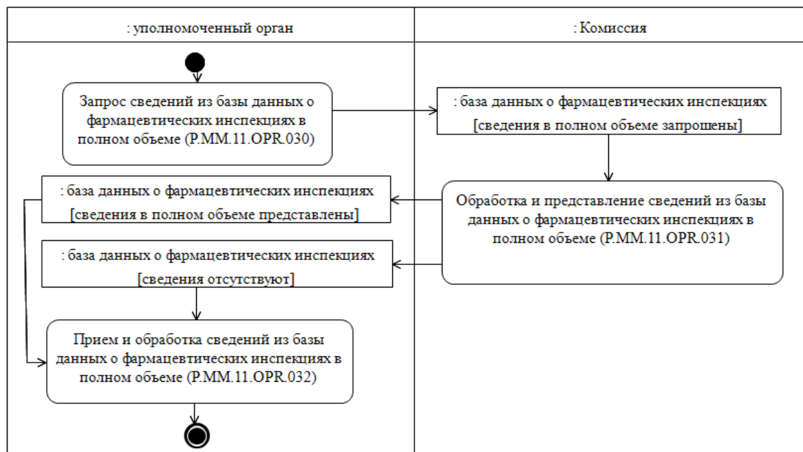
Рис. 14. Схема выполнения процедуры «Получение сведений из базы данных о фармацевтических инспекциях в полном объеме» (P.MM.11.PRC.010)
