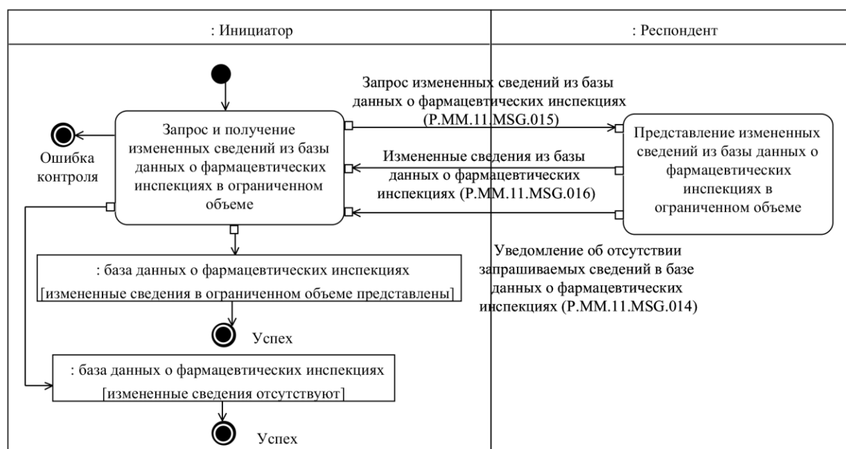
Рис. 5. Схема выполнения транзакции общего процесса «Получение измененных сведений из базы данных о фармацевтических инспекциях в ограниченном объеме» (P.MM.11.TRN.014)
