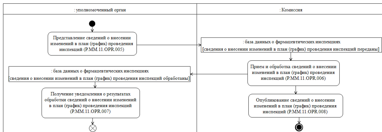
Рис. 6. Схема выполнения процедуры «Представление в Комиссию сведений о внесении изменений в план (график) проведения инспекций» (Р.ММ.11.PRC.002)
