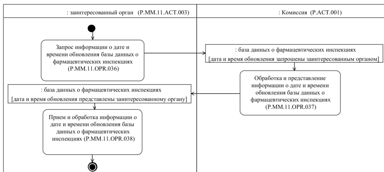
Рис. 16. Схема выполнения процедуры «Получение информации о дате и времени обновления базы данных о фармацевтических инспекциях заинтересованным органом» (P.MM.11.PRC.012)
