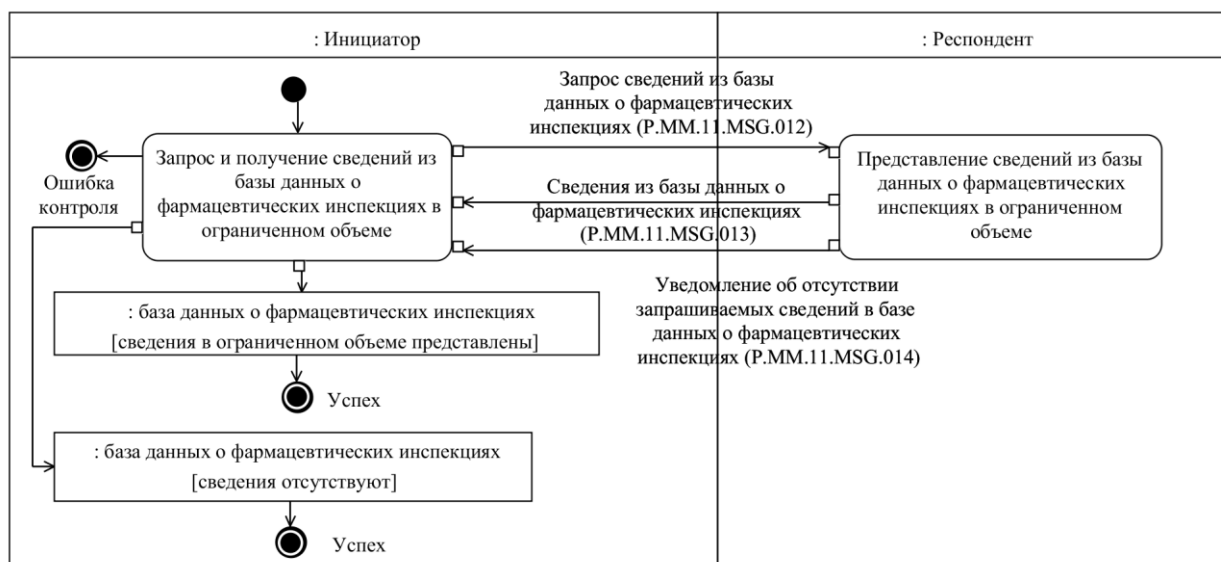
Рис. 4. Схема выполнения транзакции общего процесса «Получение сведений из базы данных о фармацевтических инспекциях в ограниченном объеме» (P.MM.11.TRN.013)
