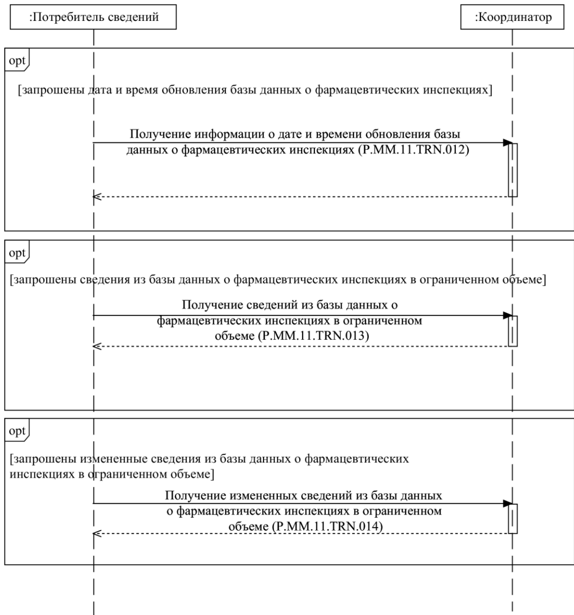
Рис. 2. Схема выполнения транзакций общего процесса при представлении сведений из базы данных о фармацевтических инспекциях
