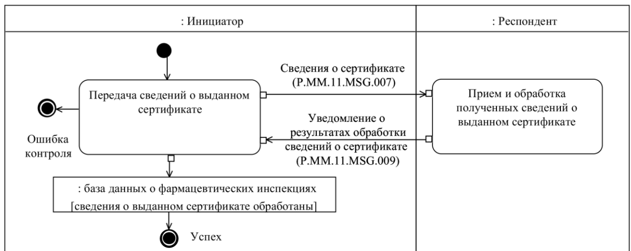
Рис. 8. Схема выполнения транзакции общего процесса «Представление сведений о выданном по результатам фармацевтической инспекции сертификате» (P.MM.11.TRN.005)
