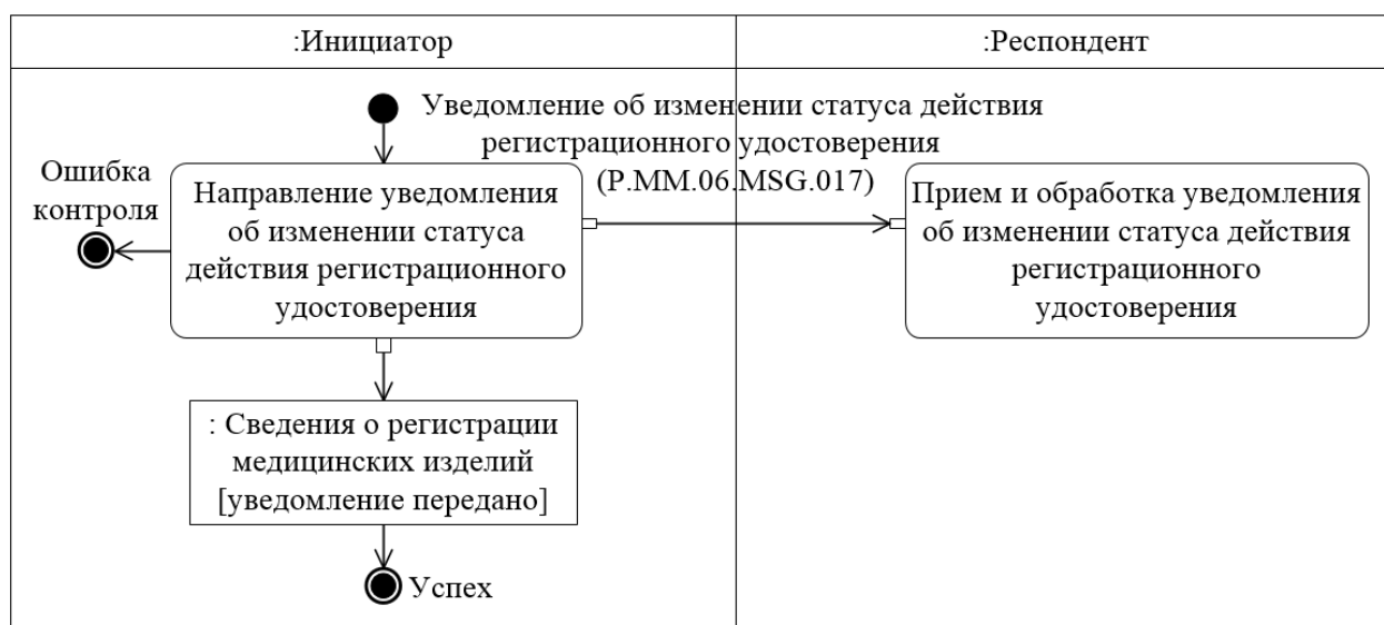
Рис. 6. Схема выполнения транзакции общего процесса «Направление уведомления об изменении статуса действия регистрационного удостоверения» (P.MM.06.TRN.008)
