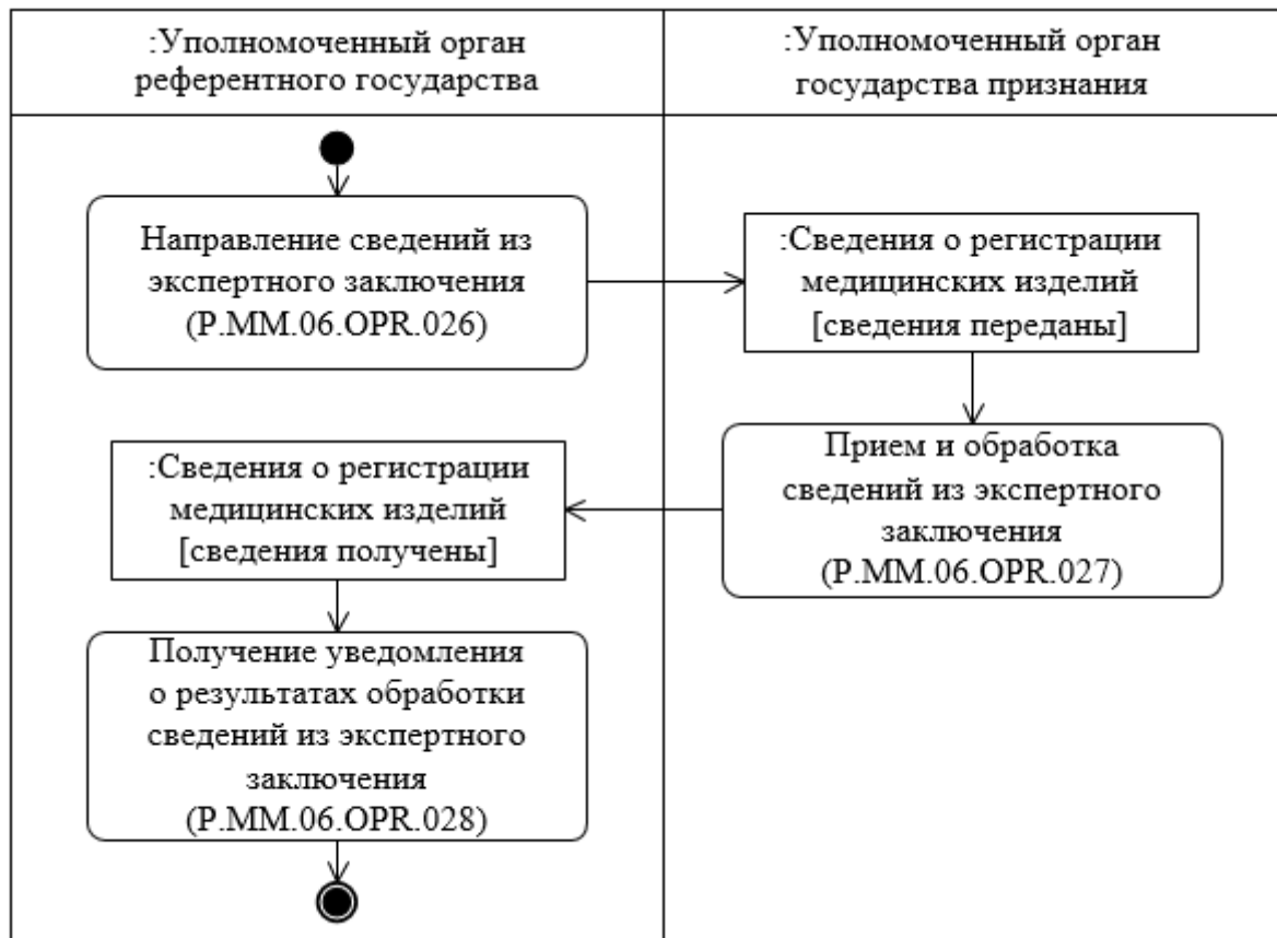
Рис. 16. Схема выполнения процедуры «Направление сведений из экспертного заключения» (P.MM.06.PRC.009)
