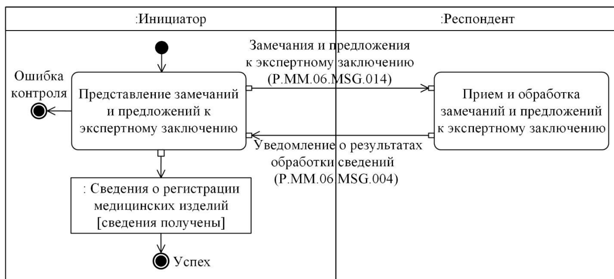
Рис. 8. Схема выполнения транзакции общего процесса «Представление замечаний и предложений к экспертному заключению» (P.MM.06.TRN.010)
