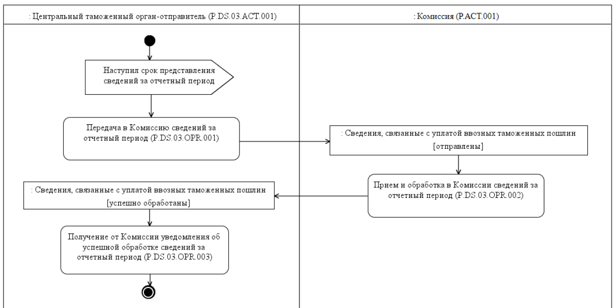
Рис. 2. Схема выполнения процедуры «Представление центральными таможенными органами в Комиссию сведений за отчетный период» (P.DS.03.PRC.001)
