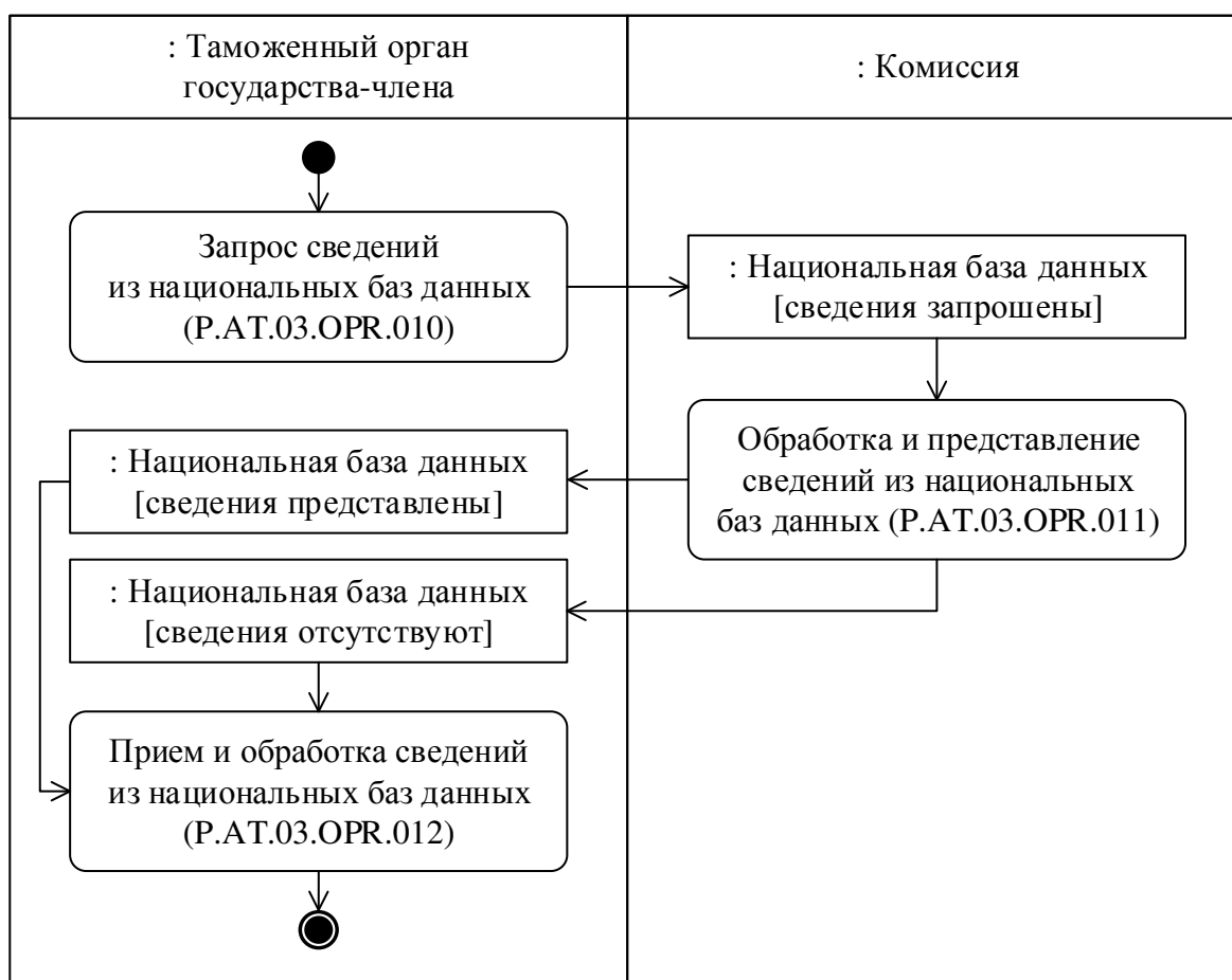
Рис. 7. Схема выполнения процедуры «Получение сведений о выданных лицензиях и (или) разрешениях» (P.AT.03.PRC.004)
