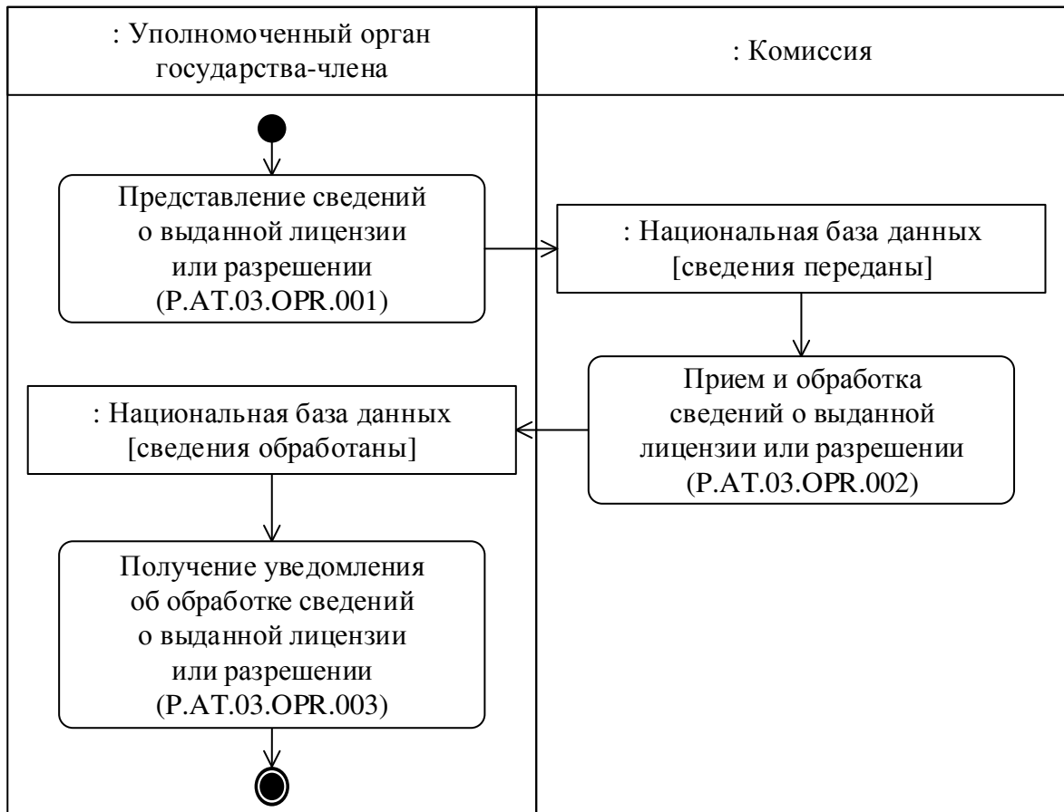
Рис. 4. Схема выполнения процедуры «Представление сведений о выданной лицензии или разрешении, включенных в национальную базу данных» (P.AT.03.PRC.001)
