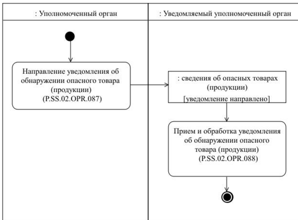
Рис. 36. Схема выполнения процедуры «Уведомление об обнаружении опасного товара (продукции)» (P.SS.02.PRC.026)
