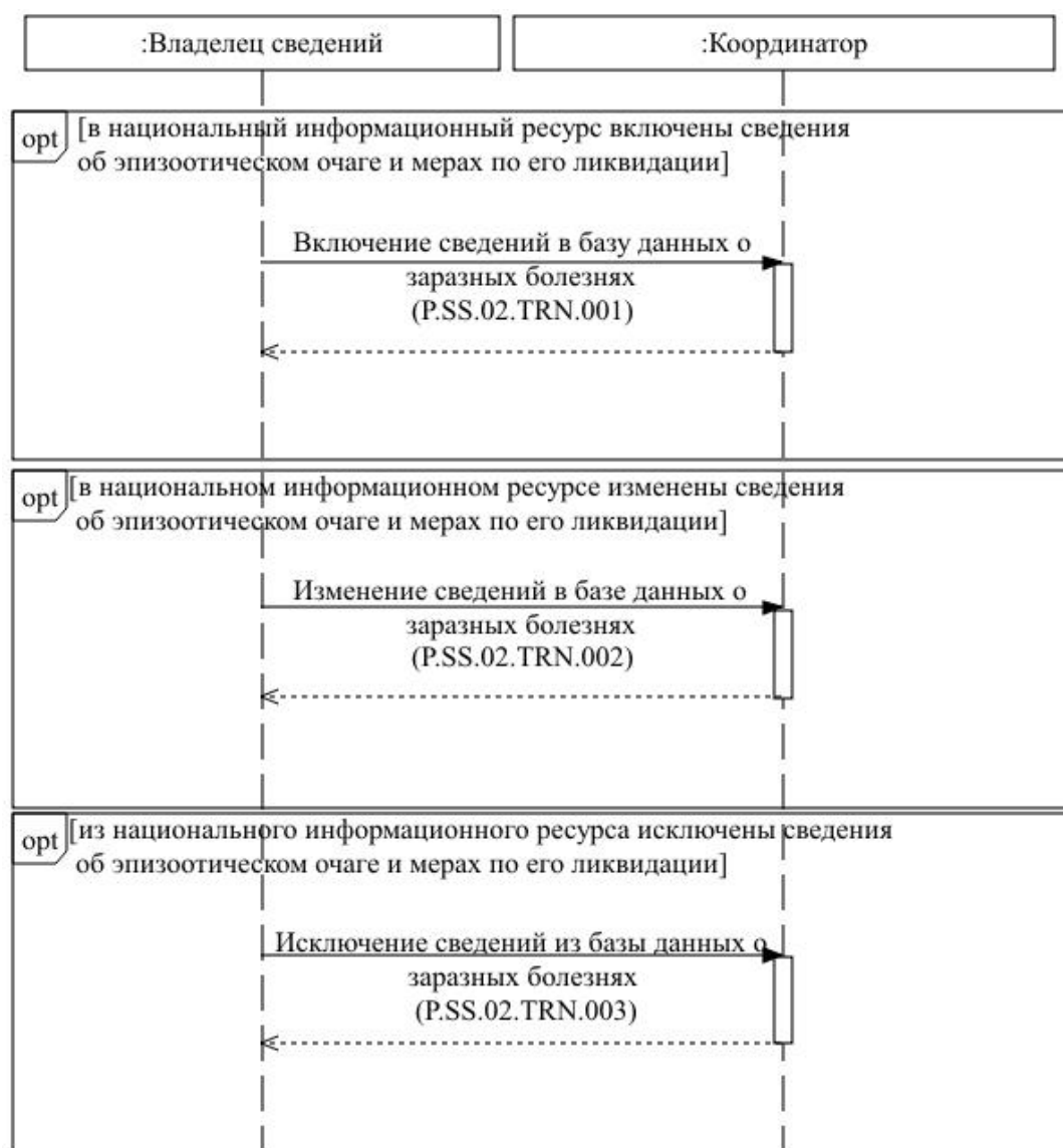
Рис. 2. Схема выполнения транзакций общего процесса при формировании и ведении базы данных о заразных болезнях
