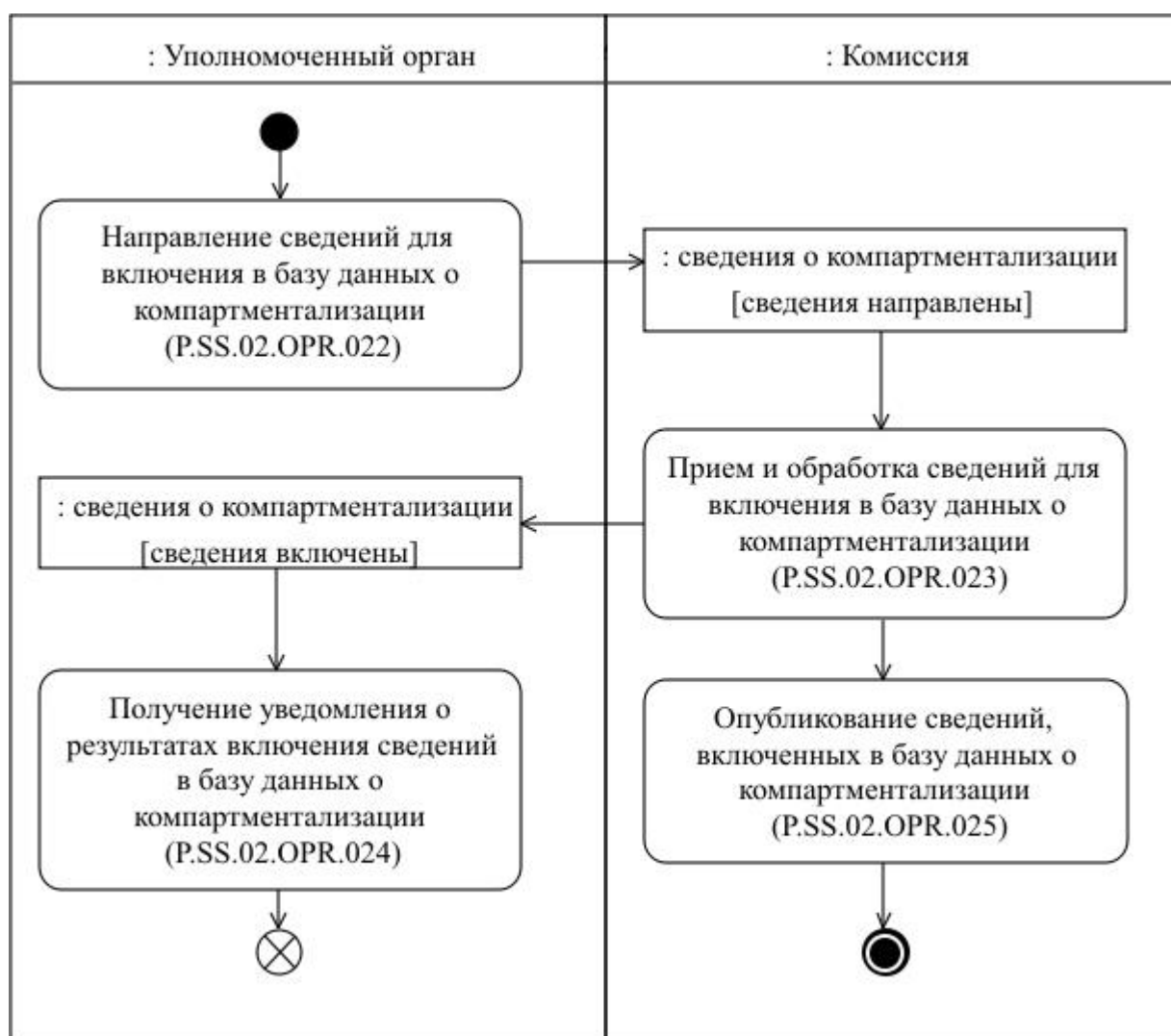
Рис. 17. Схема выполнения процедуры «Включение сведений в базу данных о компартиментализации» (P.SS.02.PRC.007)
