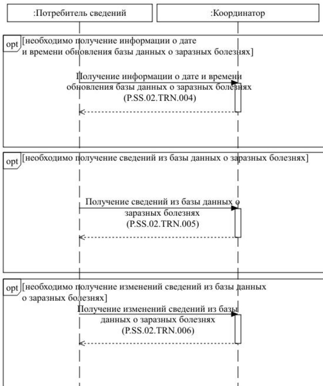
Рис. 3. Схема выполнения транзакций общего процесса при получении сведений из базы данных о заразных болезнях
