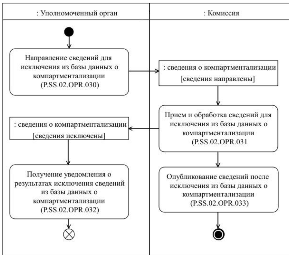
Рис. 19. Схема выполнения процедуры «Исключение сведений из базы данных о компартиментализации» (P.SS.02.PRC.009)
