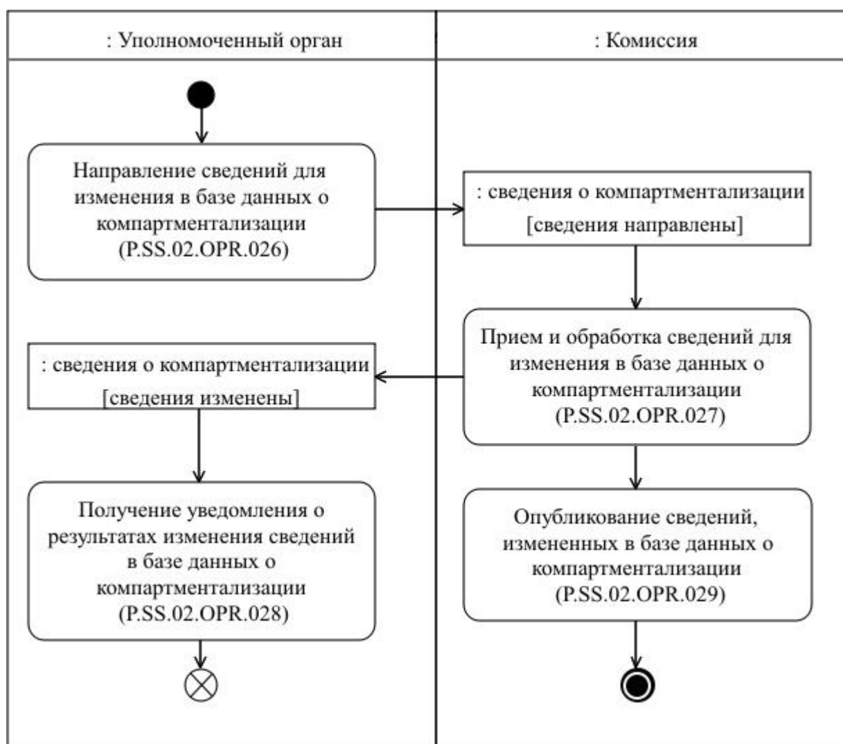
Рис. 18. Схема выполнения процедуры «Изменение сведений в базе данных о компартиментализации» (P.SS.02.PRC.008)
