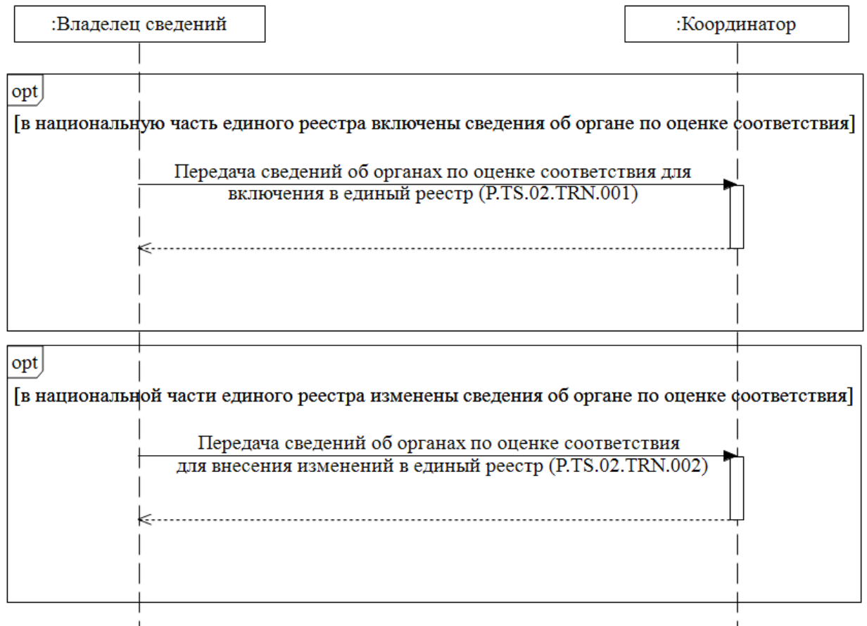
Рис. 2. Схема выполнения транзакций общего процесса при формировании и ведении единого реестра
