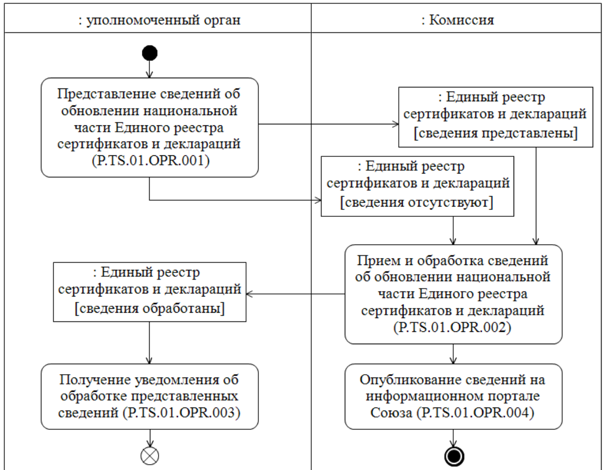
Рис. 2. Схема выполнения процедуры «Представление сведений об обновлении национальной части Единого реестра сертификатов и деклараций» (P.TS.01.PRC.001)
