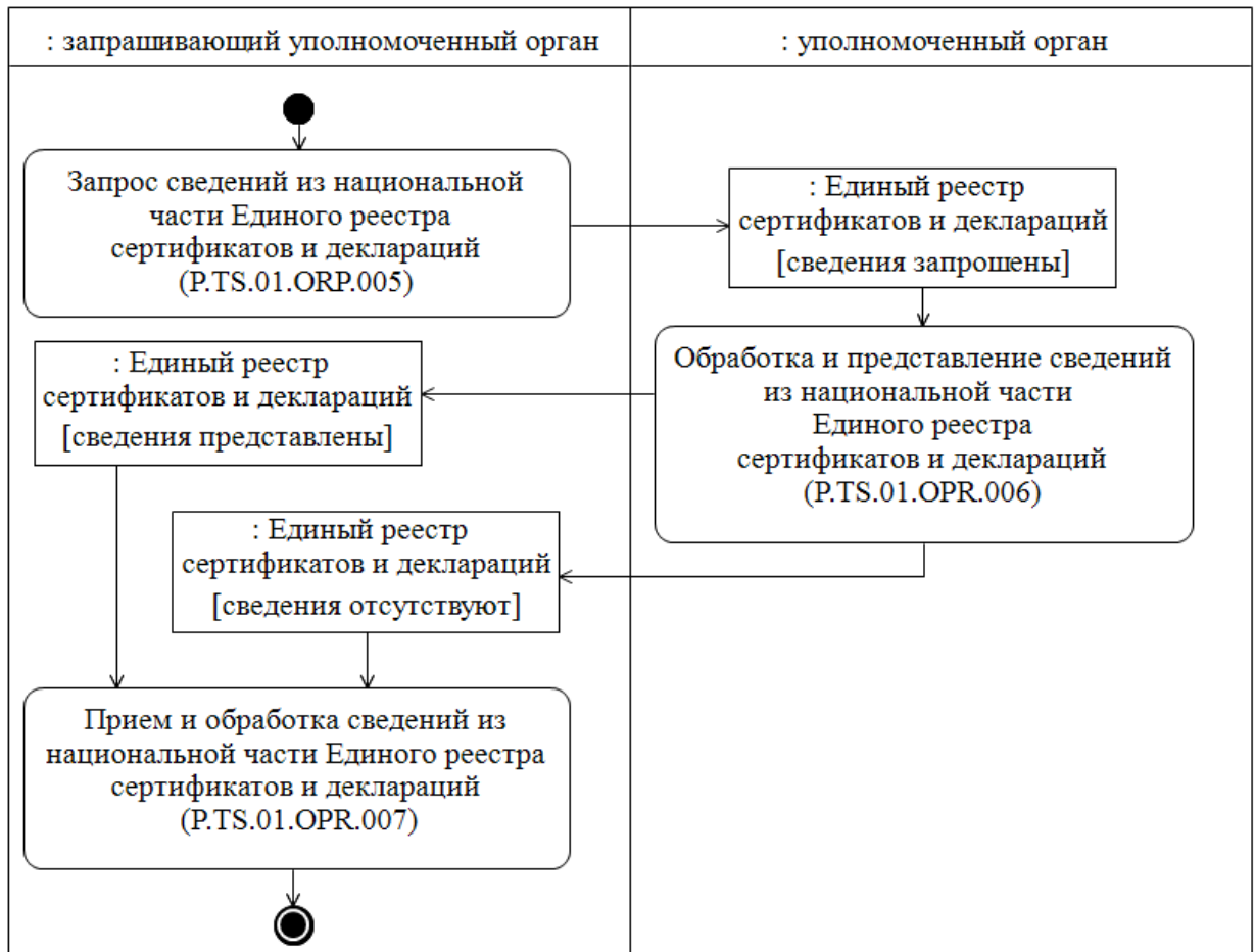
Рис. 3. Схема выполнения процедуры «Получение сведений из национальной части Единого реестра сертификатов и деклараций» (P.TS.01.PRC.002)
