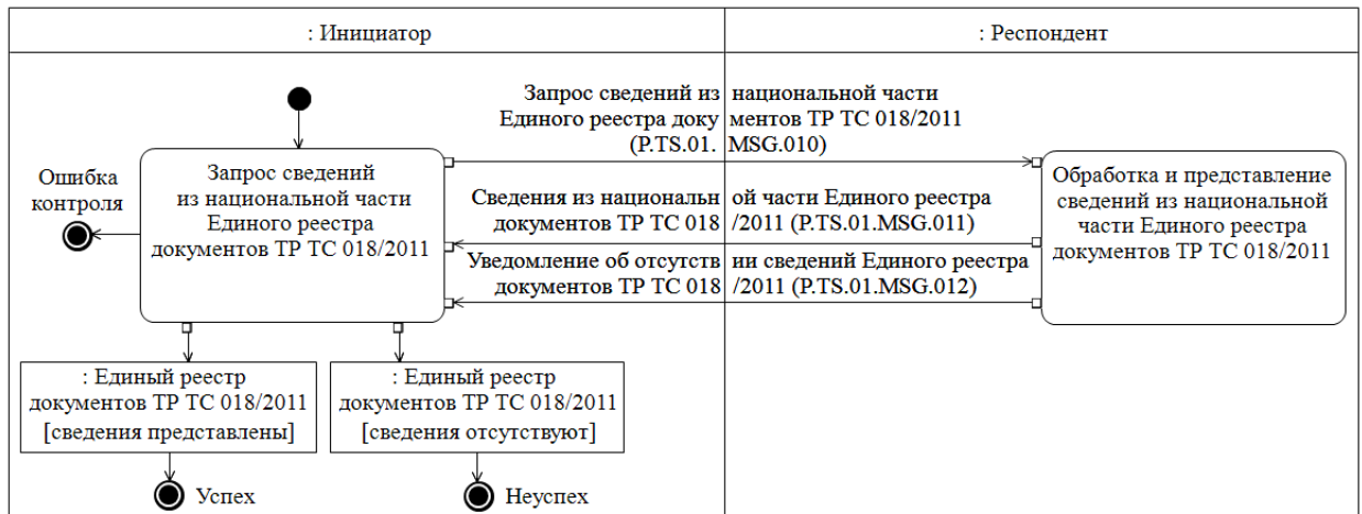
Рис. 3. Схема выполнения транзакции общего процесса «Получение сведений из национальной части Единого реестра документов ТР ТС 018/2011» (P.TS.01.TRN.006)
