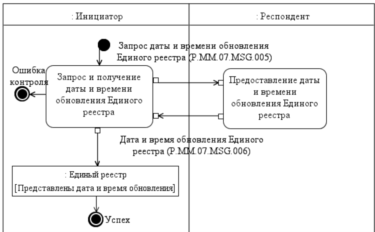
Рис. 7. Схема выполнения транзакции общего процесса «Получение даты и времени обновления Единого реестра» (P.MM.07.TRN.004)
