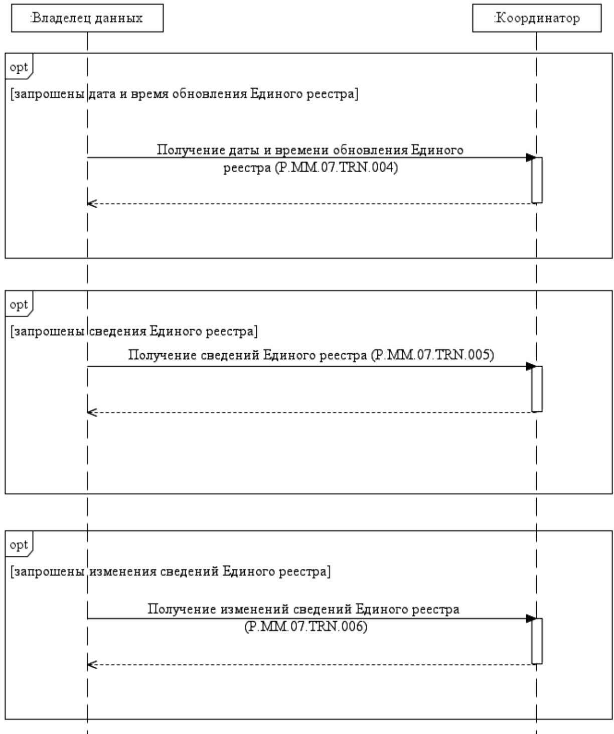
Рис. 3. Схема выполнения транзакций общего процесса при использовании Единого реестра
