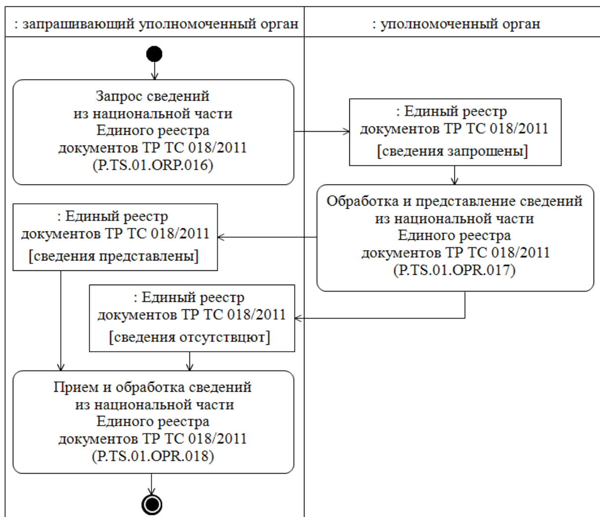
Рис. 4. Схема выполнения процедуры «Получение сведений из национальной части Единого реестра документов ТР ТС 018/2011» (P.TS.01.PRC.005)
