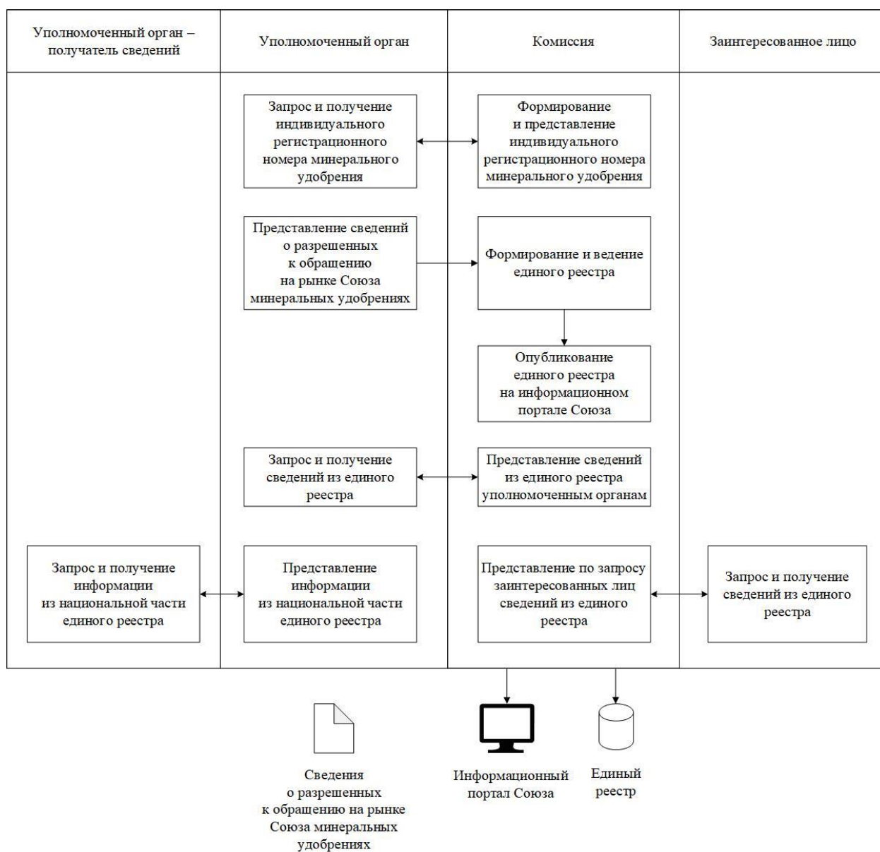
Рис. 1. Функциональная схема информационного взаимодействия
