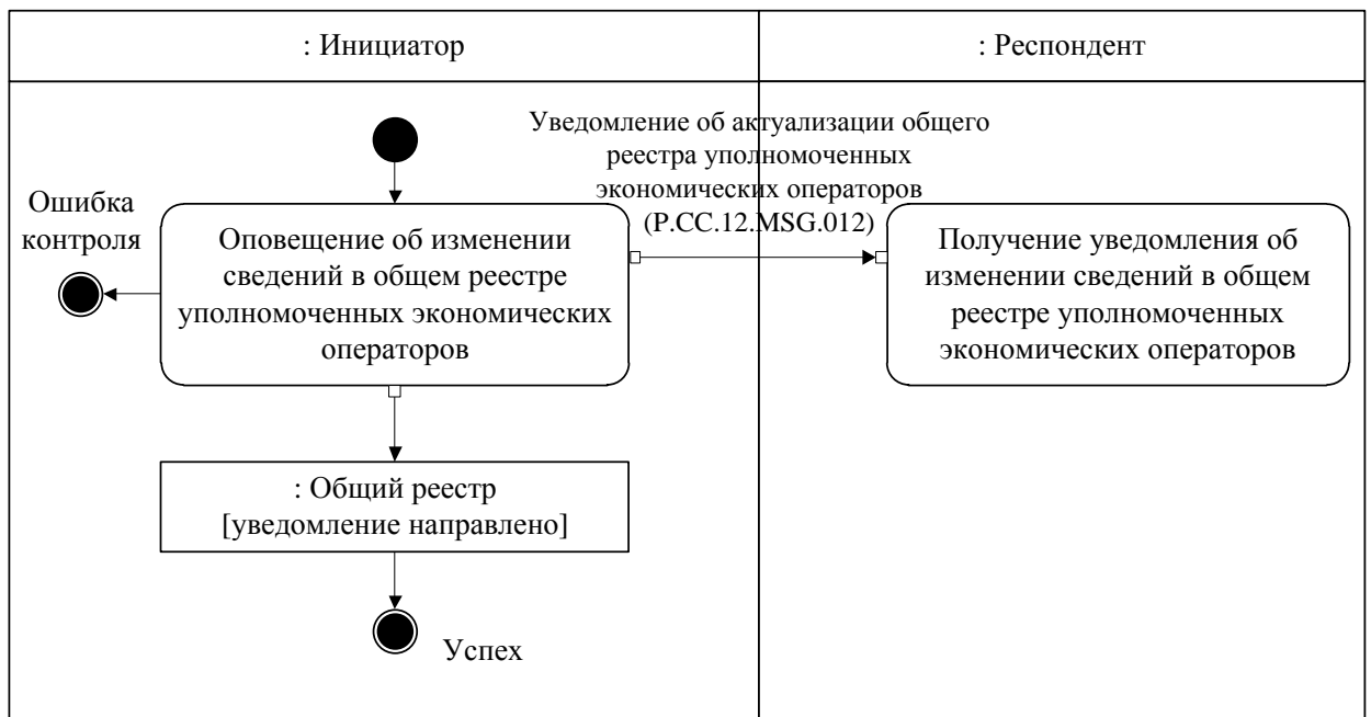
Рис. 11. Схема выполнения транзакции общего процесса «Информирование об изменении сведений в общем реестре уполномоченных экономических операторов» (P.CC.12.TRN.007)
