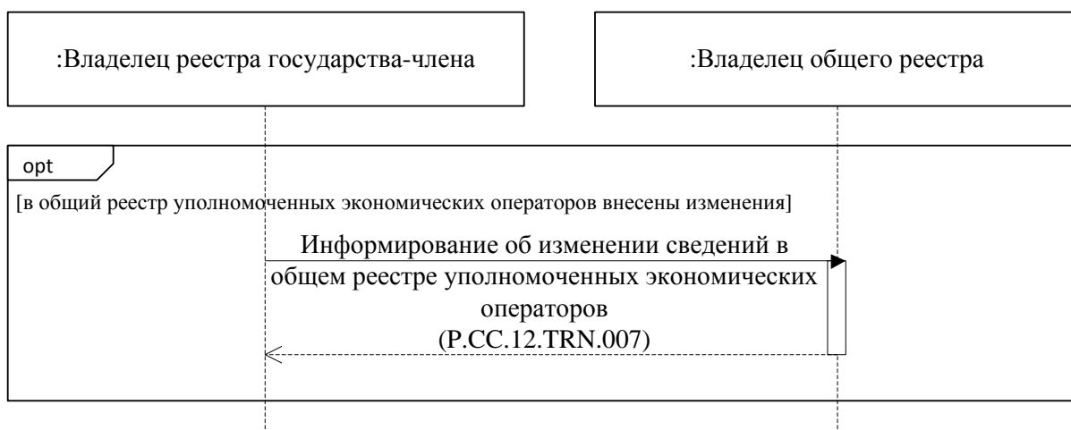
Рис. 3. Схема выполнения транзакций общего процесса при информировании об изменении сведений общего реестра уполномоченных экономических операторов
