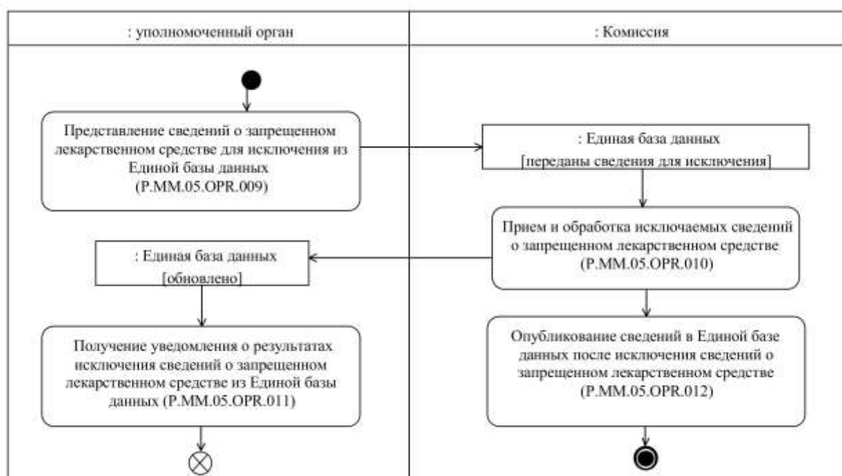
Рис. 6. Схема выполнения процедуры «Исключение сведений из Единой базы данных» (P.MM.05.PRC.003)
