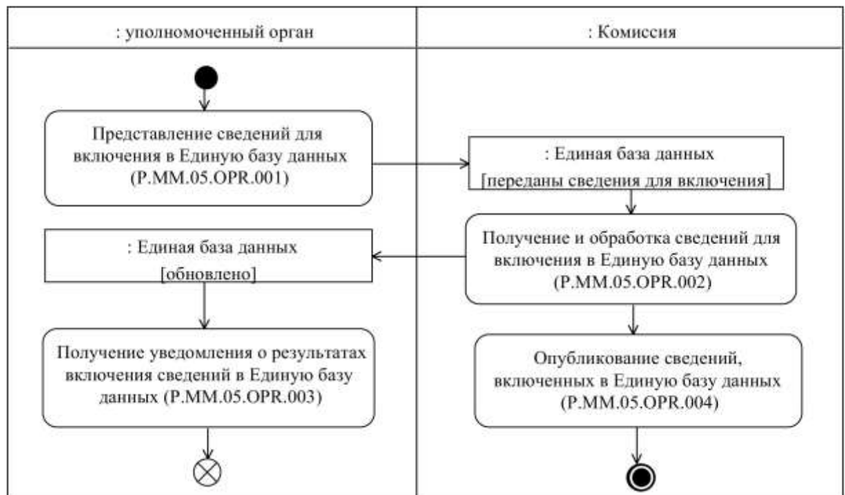
Рис. 4. Схема выполнения процедуры «Включение сведений в Единую базу данных» (P.MM.05.PRC.001)
