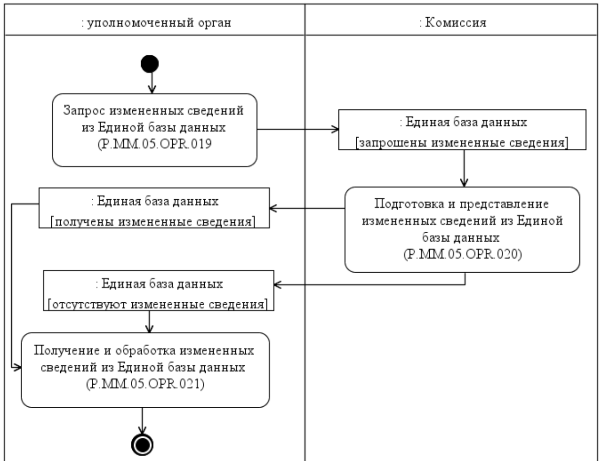
Рис. 9. Схема выполнения процедуры «Получение измененных сведений из Единой базы данных» (P.MM.05.PRC.006)
