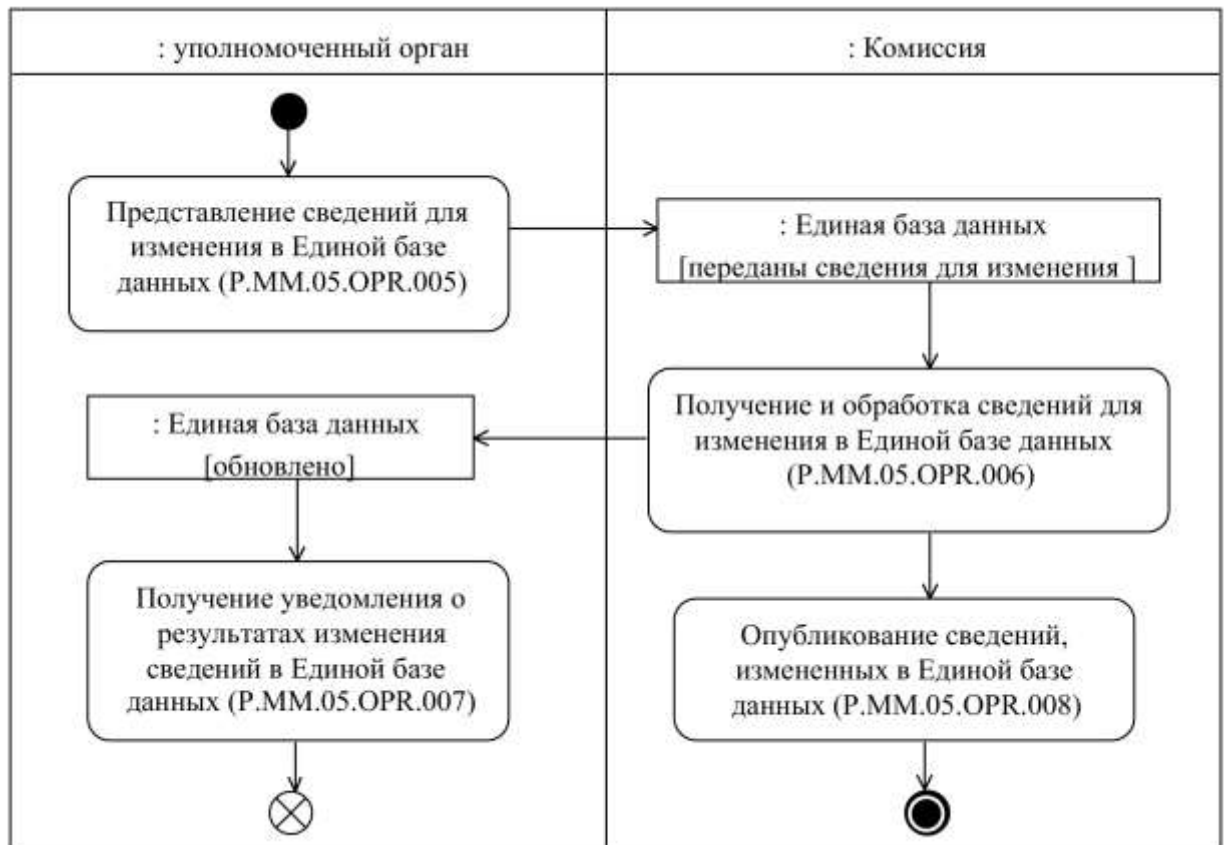
Рис. 5. Схема выполнения процедуры «Изменение сведений в Единой базе данных» (P.MM.05.PRC.002)
