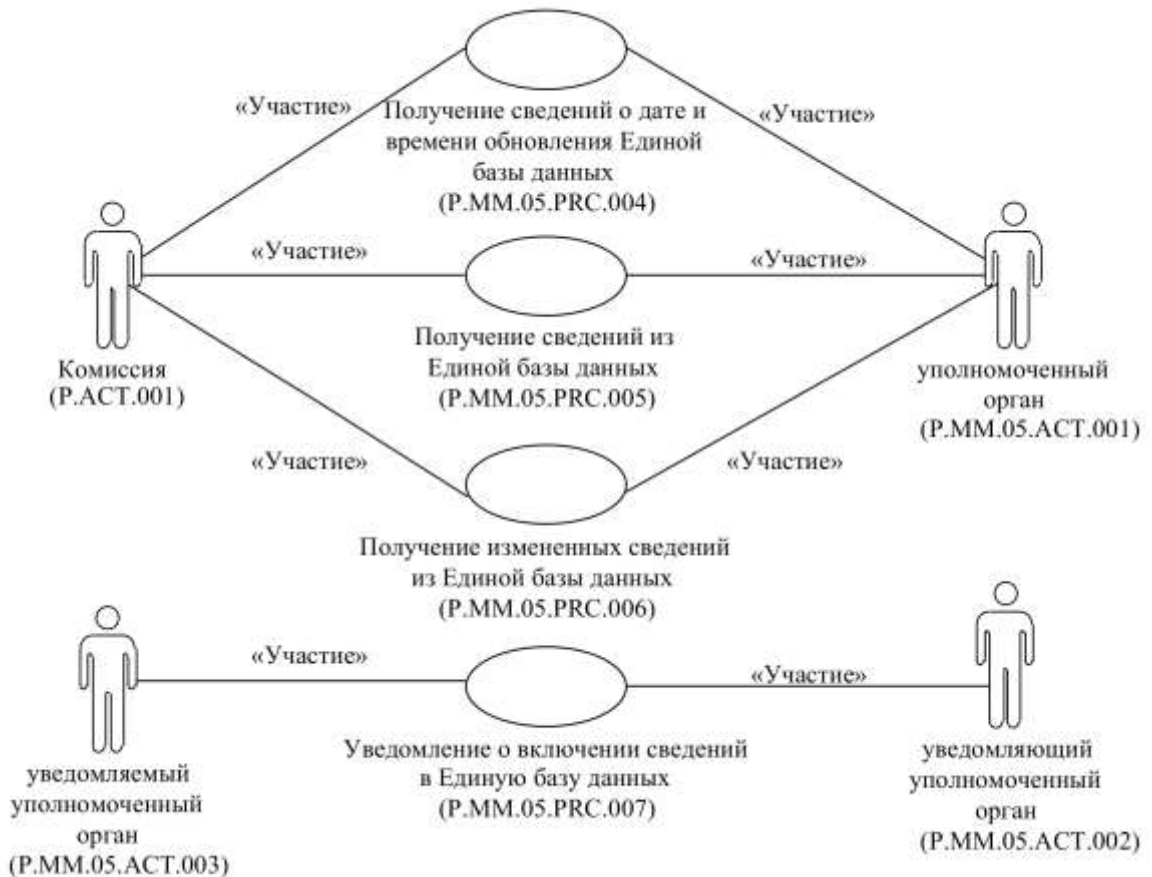
Рис. 3. Общая схема группы процедур получения сведений из Единой базы данных
