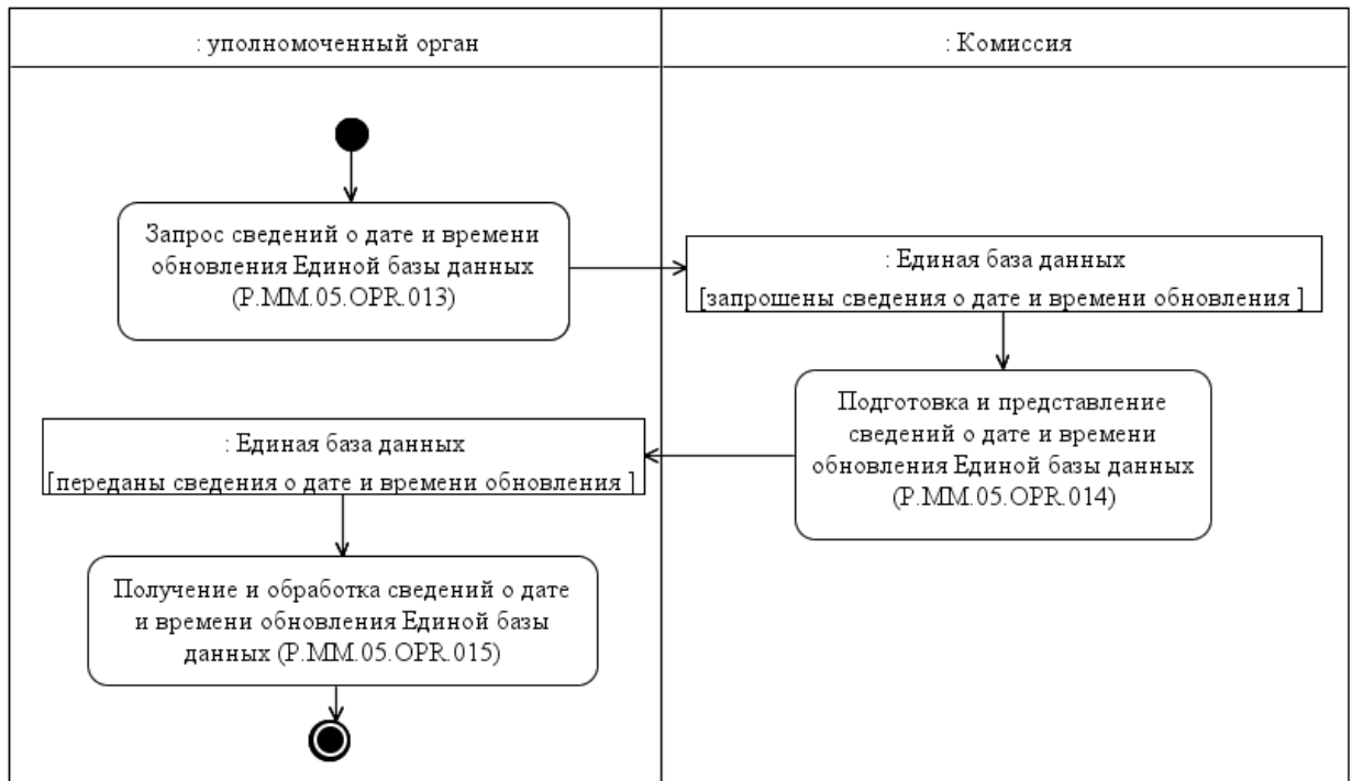
Рис. 7. Схема выполнения процедуры «Получение сведений о дате и времени обновления Единой базы данных» (P.MM.05.PRC.004)
