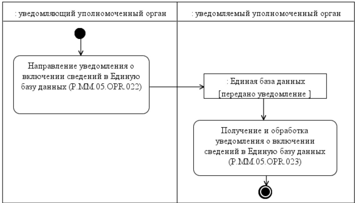
Рис. 10. Схема выполнения процедуры «Уведомление о включении сведений в Единую базу данных» (Р.ММ.05.ПРС.007)
