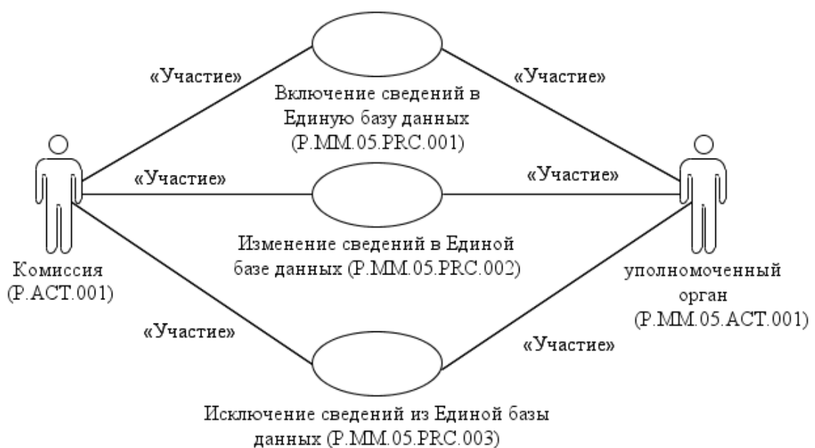
Рис. 2. Общая схема группы процедур формирования и ведения Единой базы данных
