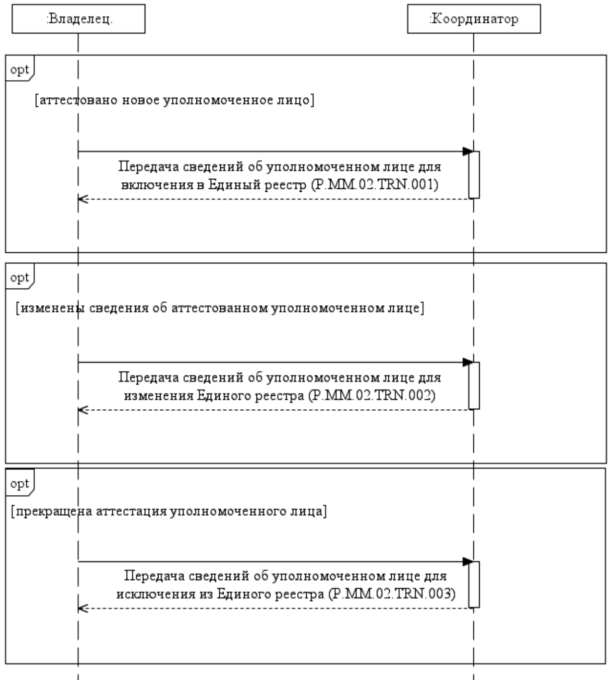
Рис. 2. Схема выполнения транзакций общего процесса при формировании и ведении Единого реестра
