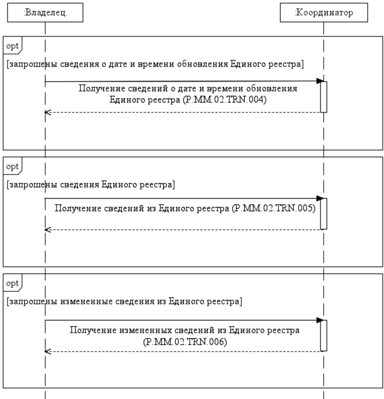
Рис. 3. Схема выполнения транзакций общего процесса при получении сведений Единого реестра
