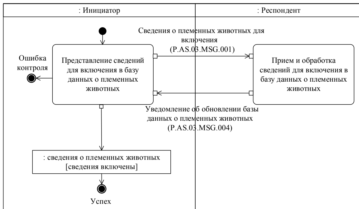
Рис. 6. Схема выполнения транзакции общего процесса «Передача сведений для включения в базу данных о племенных животных» (P.AS.03.TRN.001)
