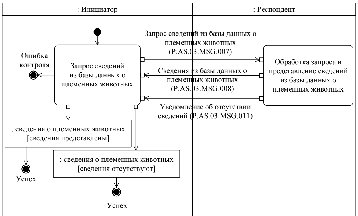
Рис. 10. Схема выполнения транзакции общего процесса «Получение сведений из базы данных о племенных животных» (P.AS.03.TRN.005)
