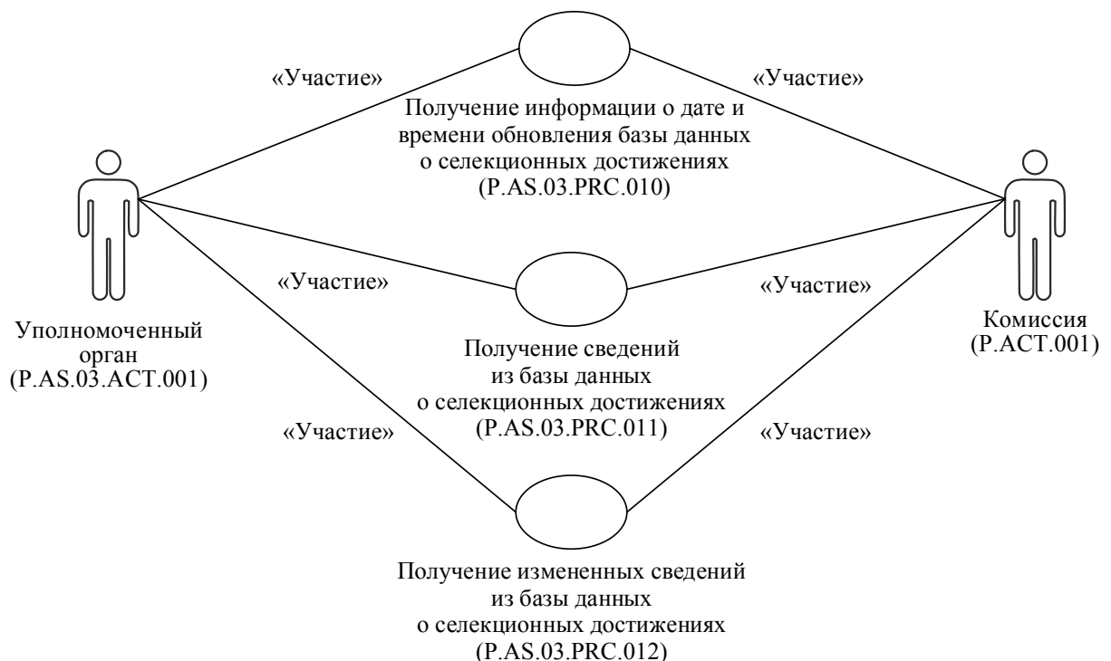
Рис. 5. Общая схема группы процедур получения сведений из базы данных о селекционных достижениях по запросу уполномоченных органов
