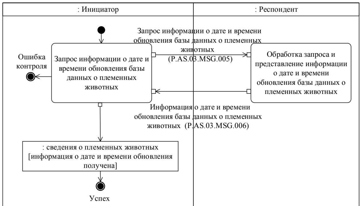
Рис. 9. Схема выполнения транзакции общего процесса «Получение информации о дате и времени обновления базы данных о племенных животных» (P.AS.03.TRN.004)
