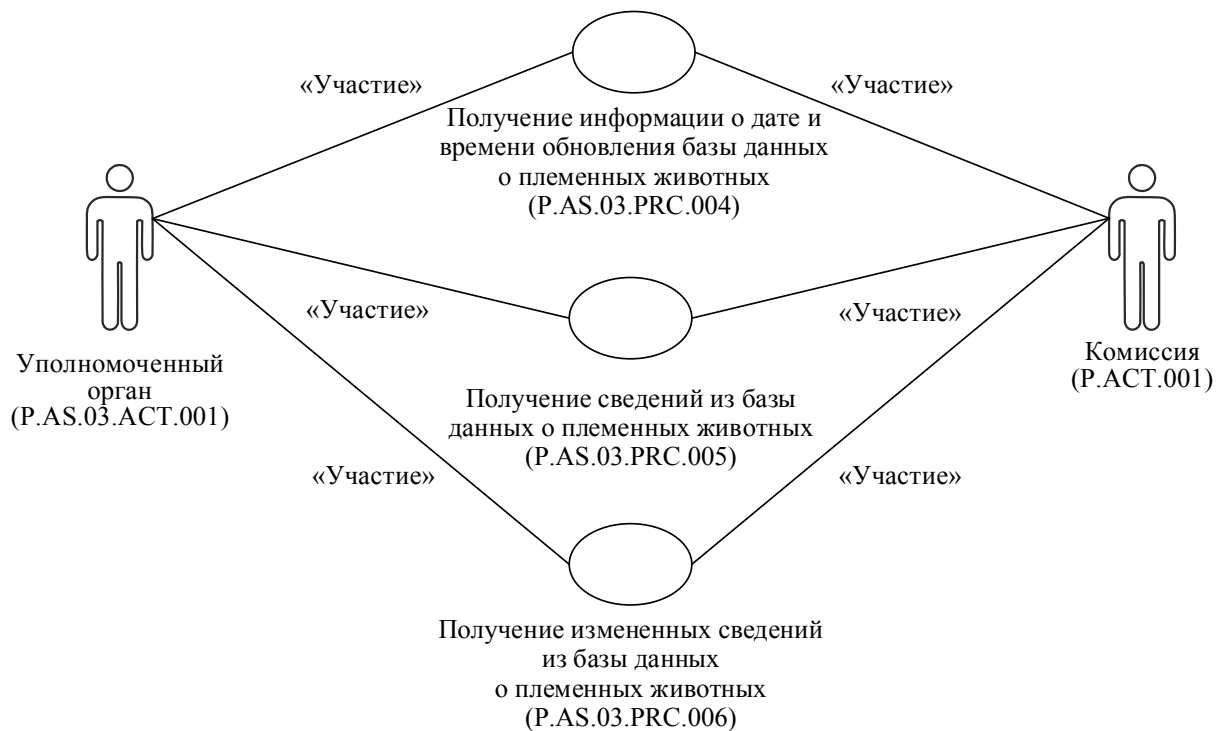
Рис. 3. Общая схема группы процедур получения сведений из базы данных о племенных животных по запросу уполномоченных органов
