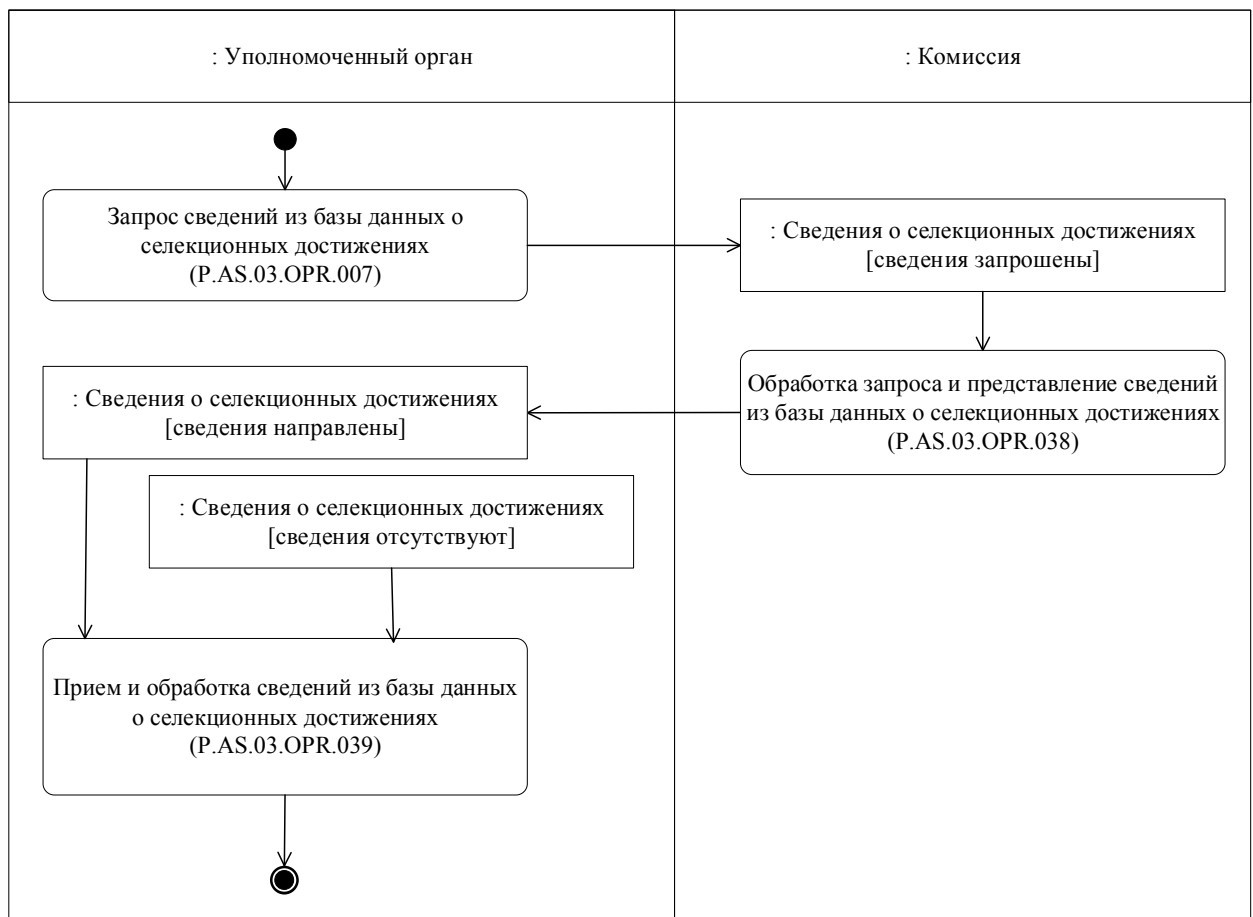
Рис. 16. Схема выполнения процедуры «Получение сведений из базы данных о селекционных достижениях» (P.AS.03.PRC.011)
