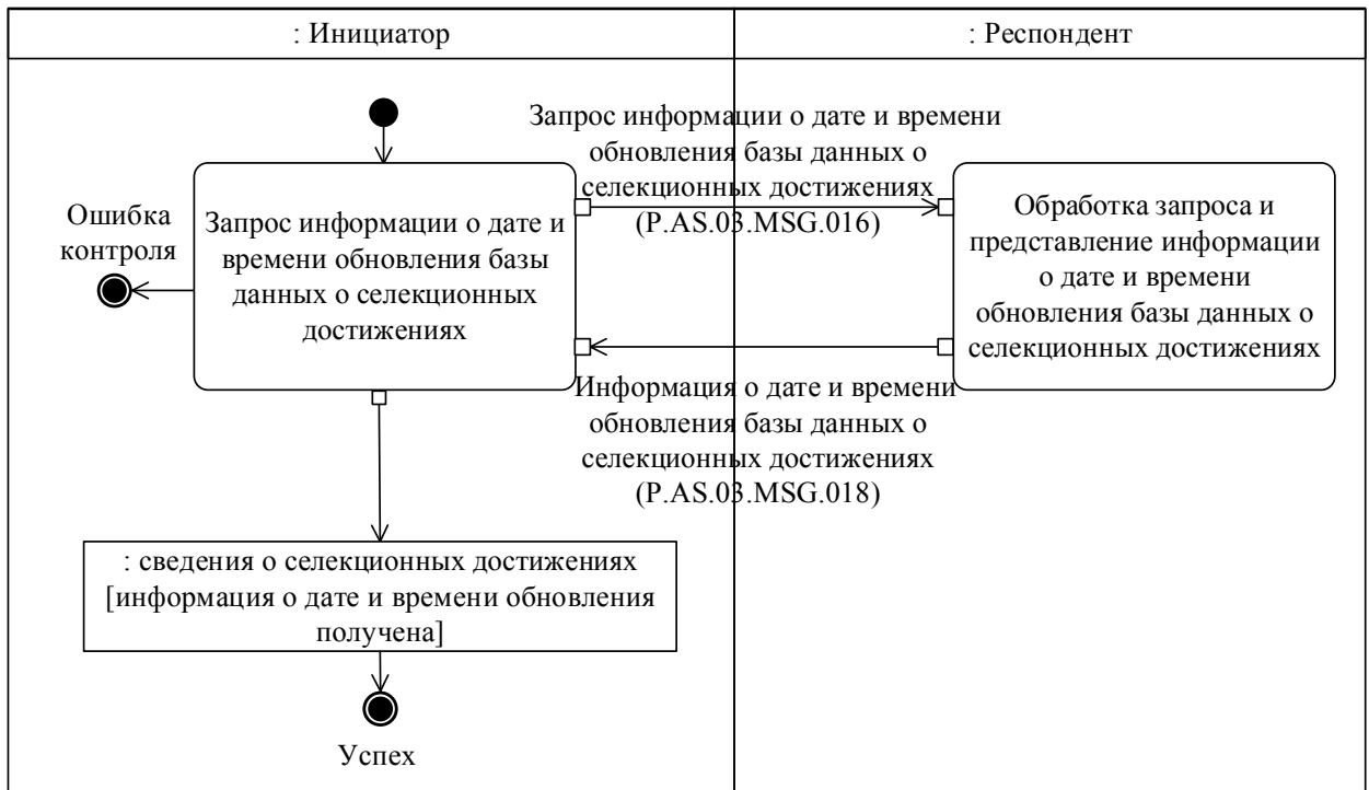
Рис. 15. Схема выполнения транзакции общего процесса «Получение информации о дате и времени обновления базы данных о селекционных достижениях» (P.AS.03.TRN.010)
