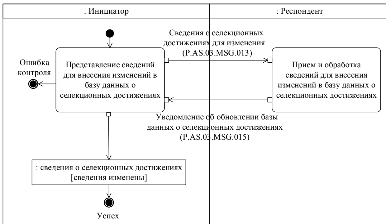
Рис. 13. Схема выполнения транзакции общего процесса «Передача сведений для внесения изменений в базу данных о селекционных достижениях» (P.AS.03.TRN.008)
