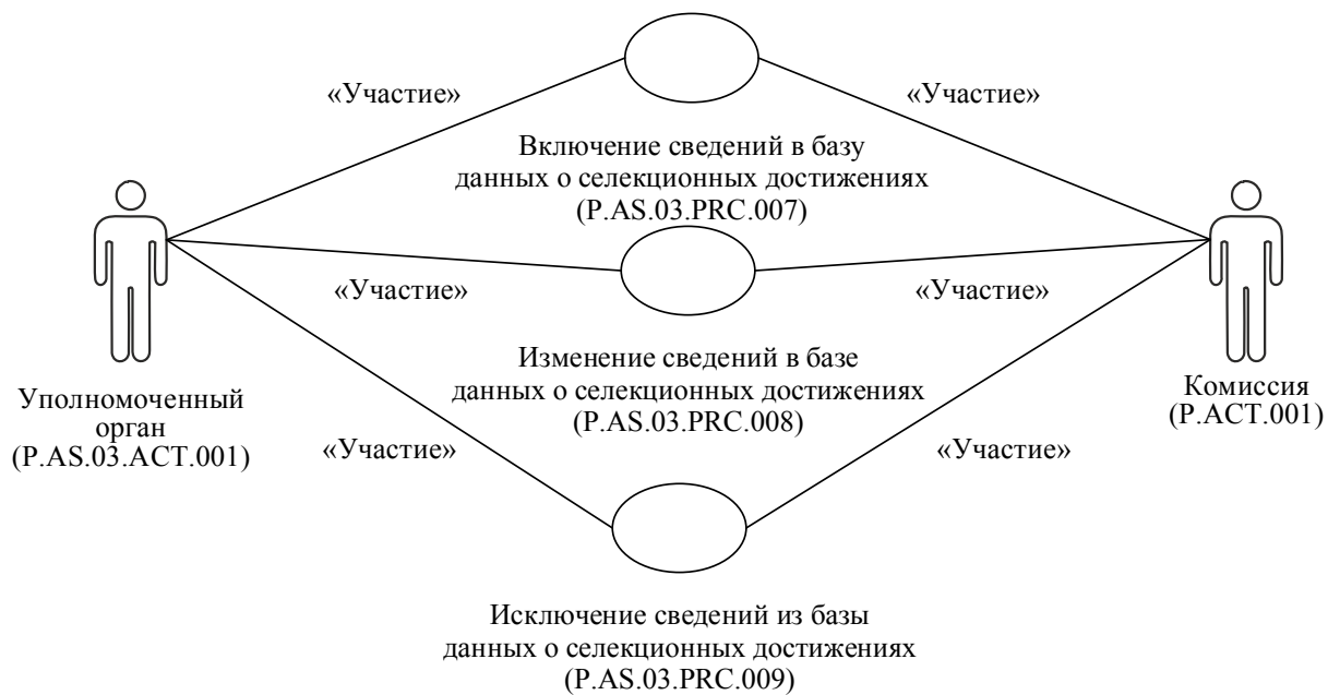
Рис. 4. Общая схема группы процедур формирования и ведения базы данных о селекционных достижениях
