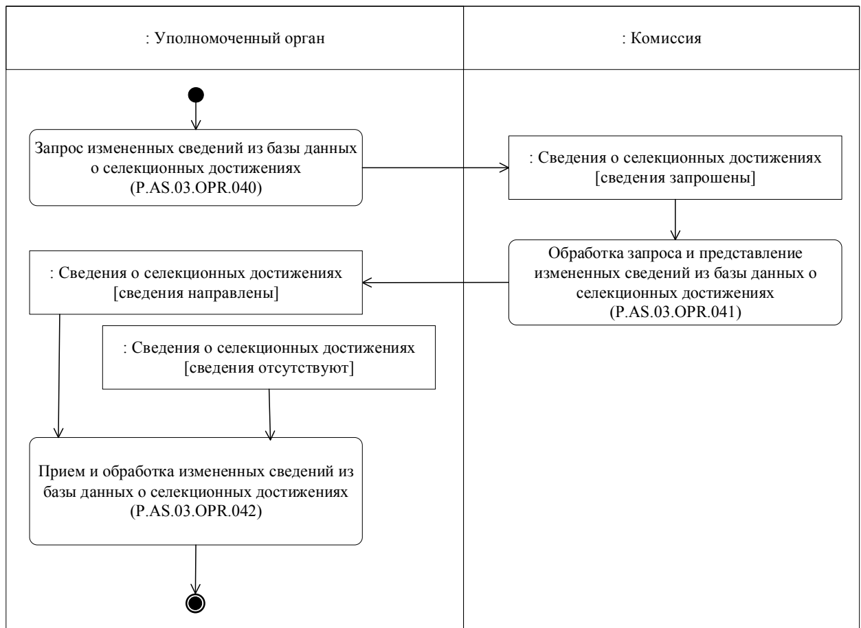
Рис. 17. Схема выполнения процедуры «Получение измененных сведений из базы данных о селекционных достижениях» (P.AS.03.PRC.012)
