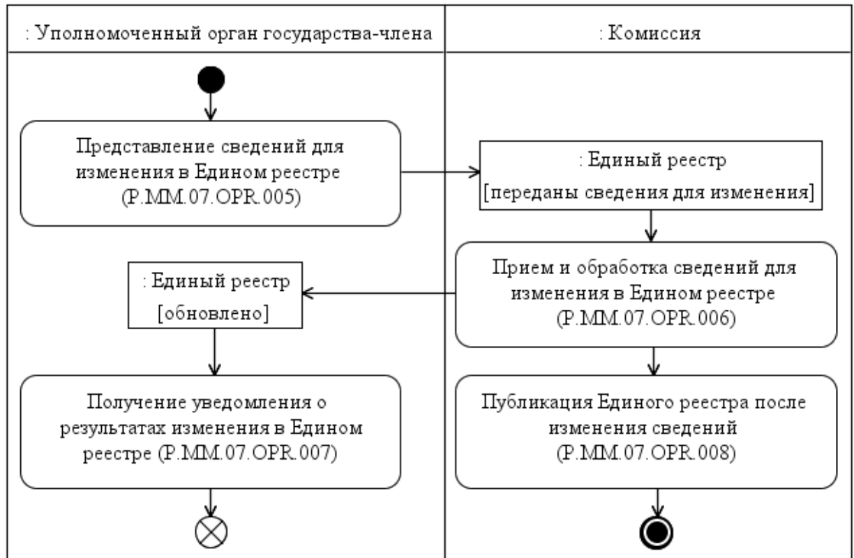
Рис. 5. Схема выполнения процедуры «Изменение сведений в Едином реестре» (P.MM.07.PRC.002)
