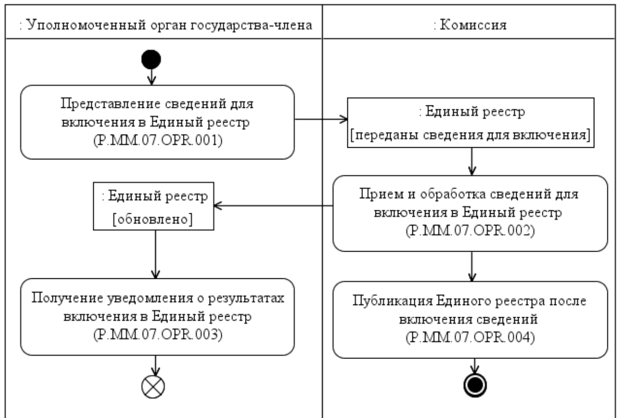
Рис. 4. Схема выполнения процедуры «Включение сведений в Единый реестр» (P.MM.07.PRC.001)
