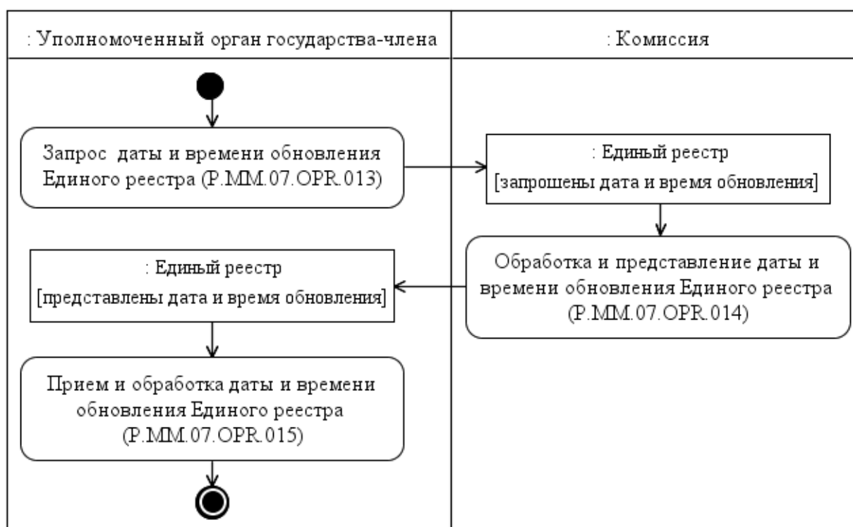
Рис. 7. Схема выполнения процедуры «Получение даты и времени обновления Единого реестра» (P.MM.07.PRC.004)
