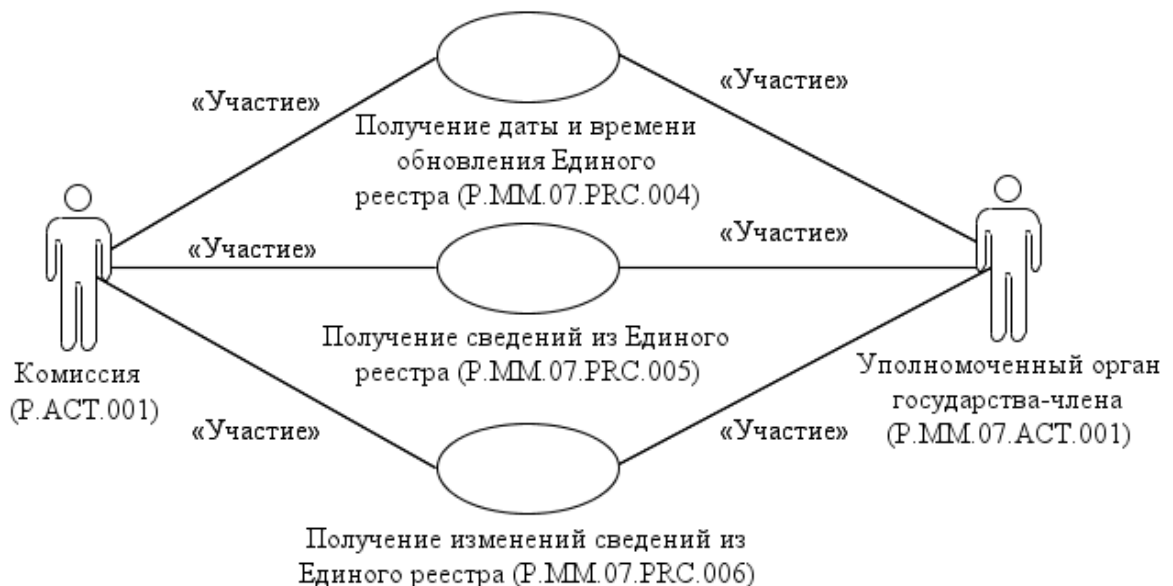
Рис. 3. Общая схема группы процедур представления сведений Единого реестра
