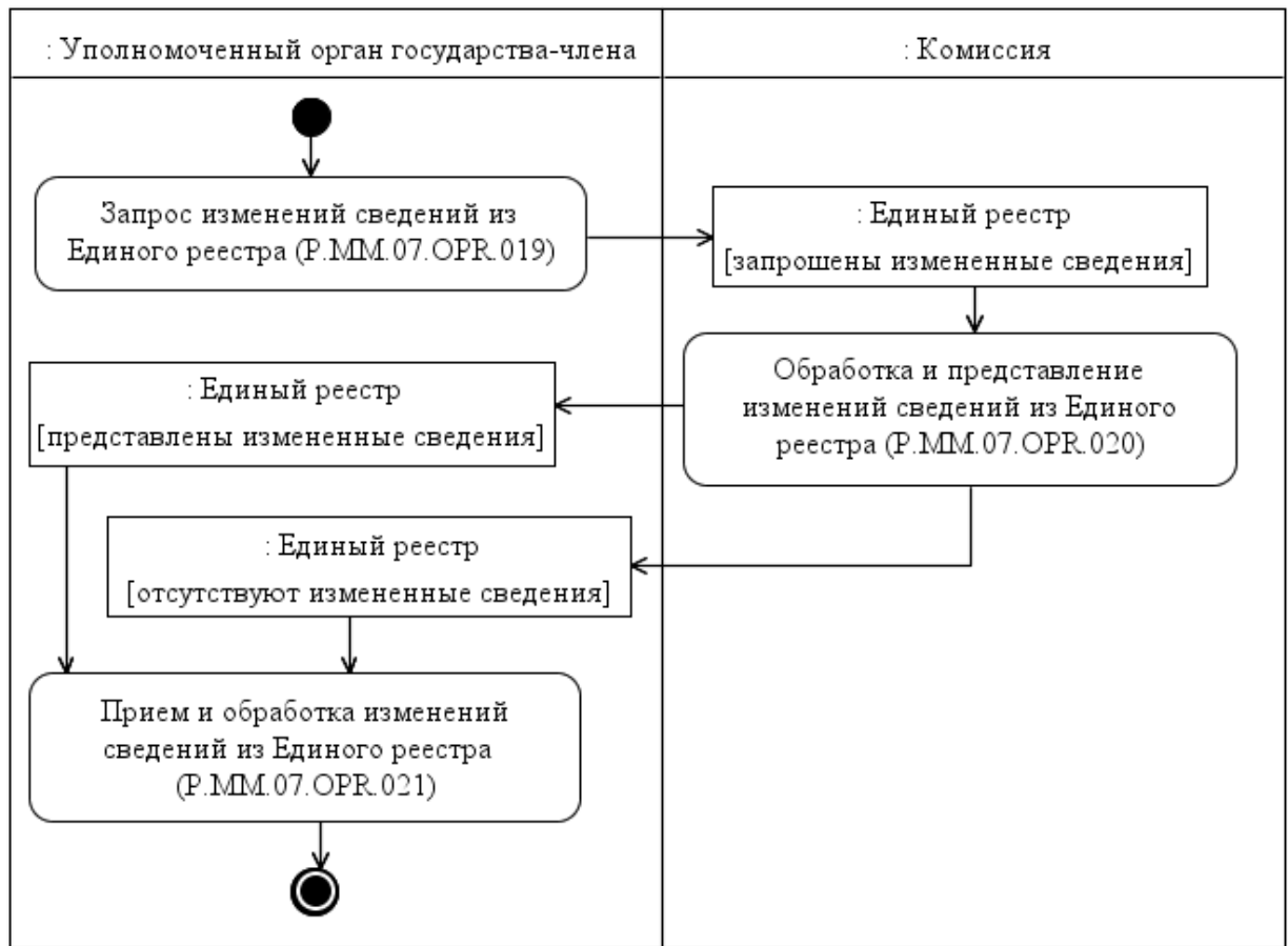
Рис. 9. Схема выполнения процедуры «Получение изменений сведений Единого реестра» (P.MM.07.PRC.006)
